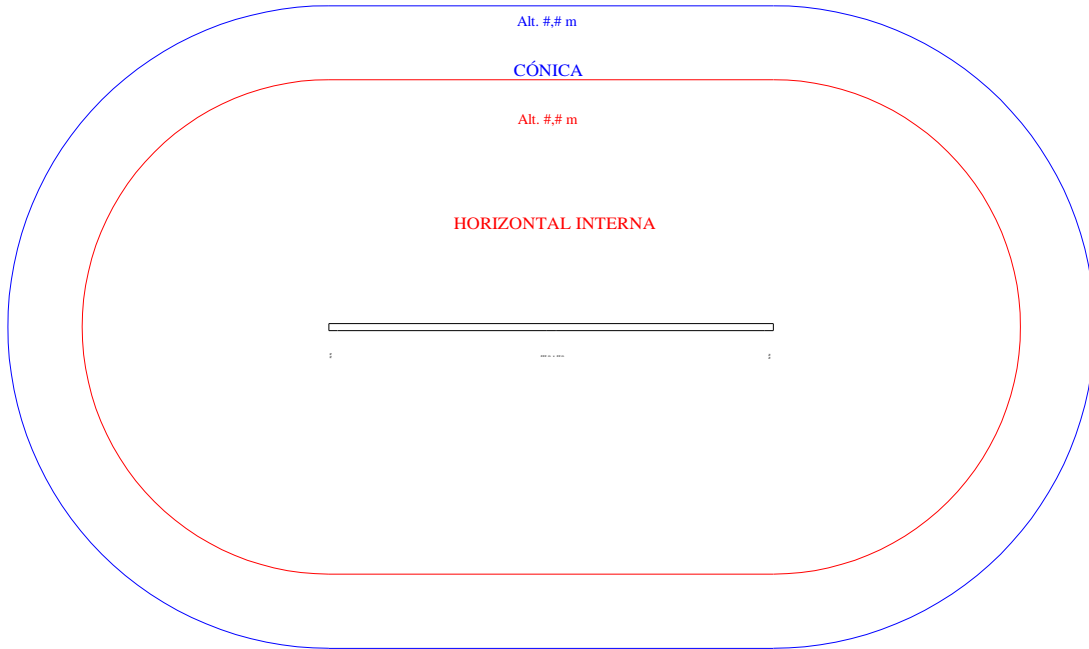
Figura 6-15- Superficie Cónica
