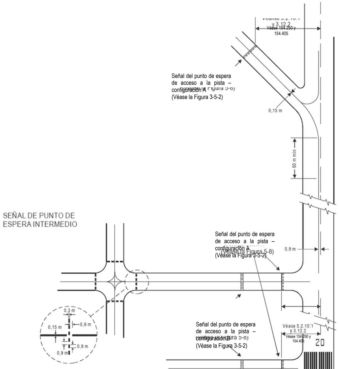
Figura 3-5-1. Grupo de señales de las calles de rodaje (indicadas junto con las señales básicas de pista)
