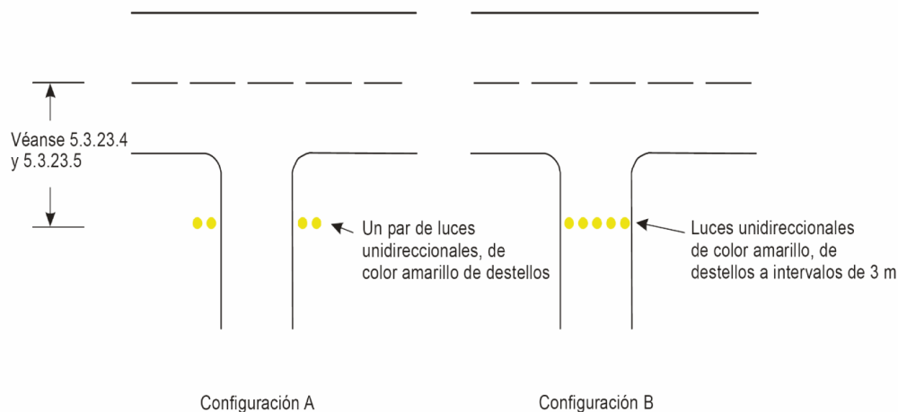
Figura 1-31-1. Luces de protección de pista
