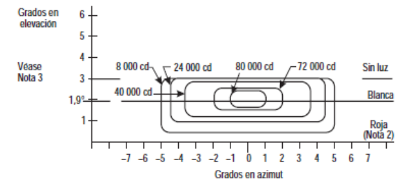
DIAGRAMA DE INDICACIÓN "ASCIENDA" DEL T-VASIS (DE DÍA)
