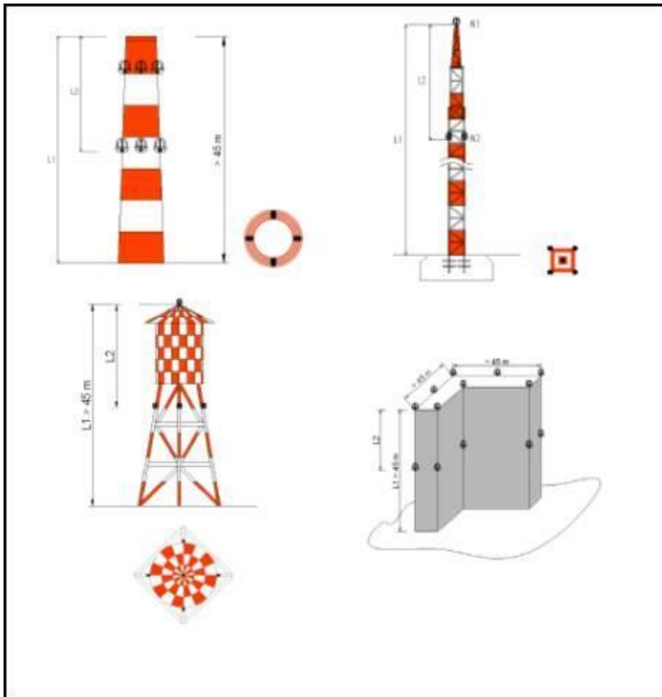
Figura 2-3-5. Ejemplos de iluminación de obstáculos/estructuras &gt;45m
