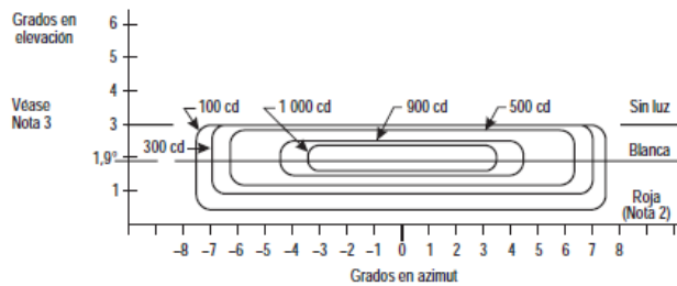
DIAGRAMA DE INDICACIÓN "ASCIENDA" DEL T-VASIS (DE NOCHE)
