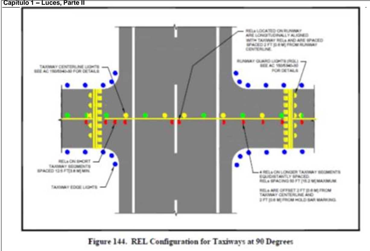
Figura 1-41-2 Sistema REL en ángulo 90°
