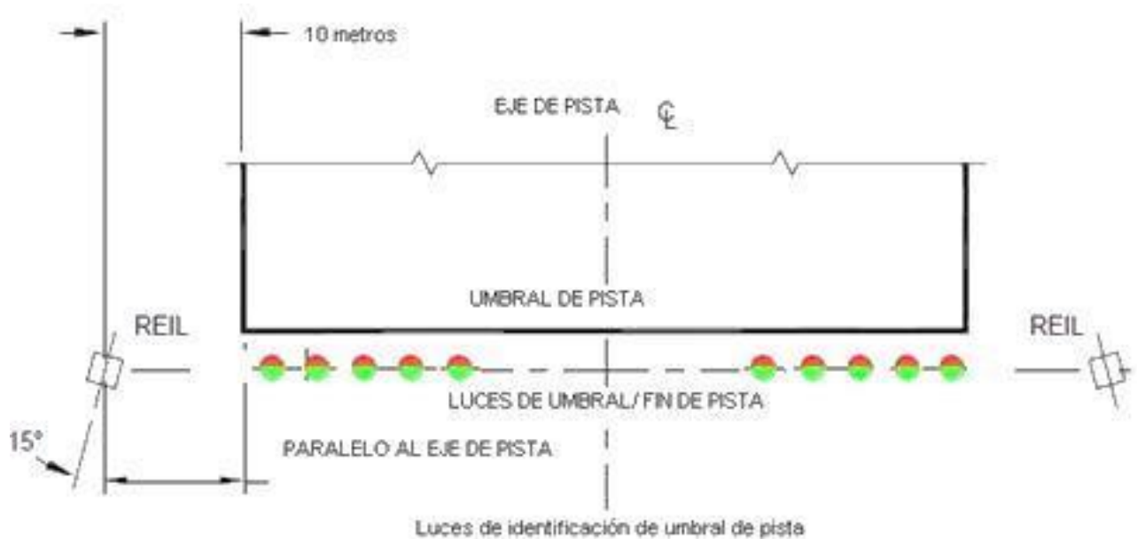
Figura 1-13-1. Luces de Identificación de umbral de pista
