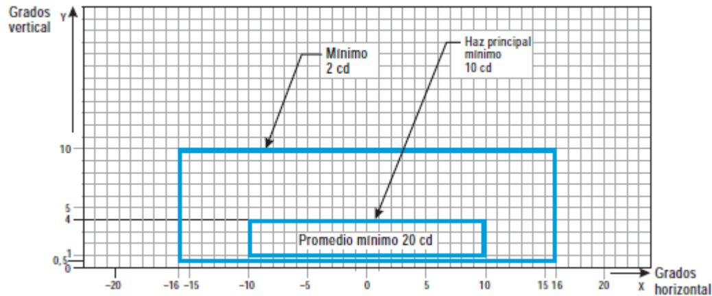
Figura ADJB-15. Diagrama de isocandelas para luces de eje de calle de rodaje (espaciado de 30 m, 60 m), de barra de prohibición de acceso y de barra de parada en tramos rectos previstas para ser utilizadas en condiciones de alcance visual en la pista de 350 m o superior
