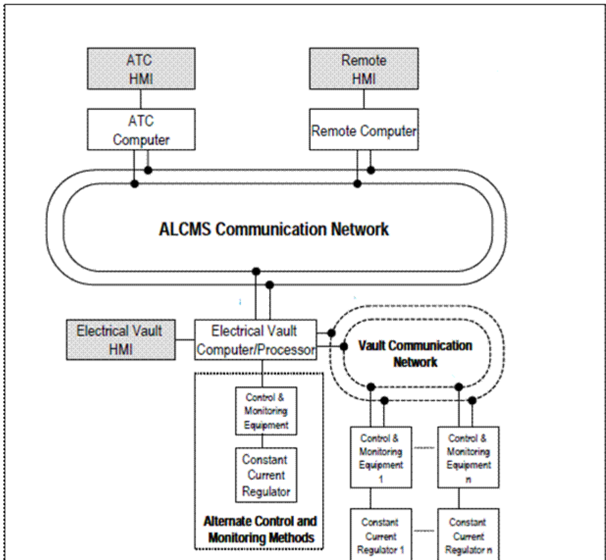
Figura ADJL-3: ALCMS Diagrama general de los Componentes
