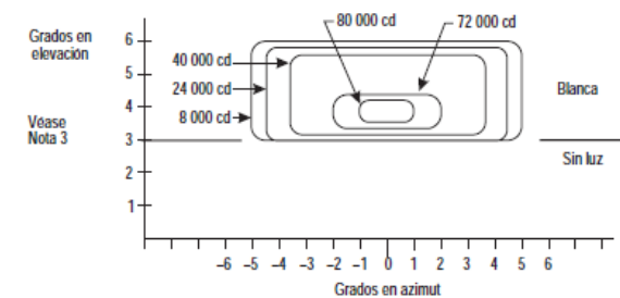
DIAGRAMA DE INDICACIÓN "DESCIENDA" DEL T-VASIS (DE DÍA)
