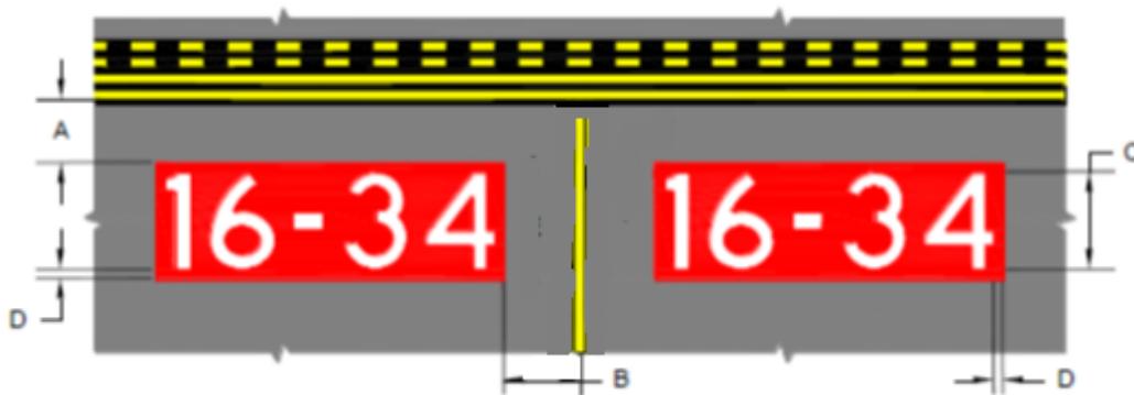
Figura 4-2-3. Dimensiones Señal con instrucciones obligatorias
