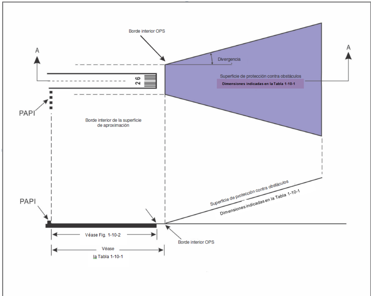
Figura 1-10-3. Superficie de protección contra obstáculos para los sistemas visuales indicadores de pendiente de aproximación
