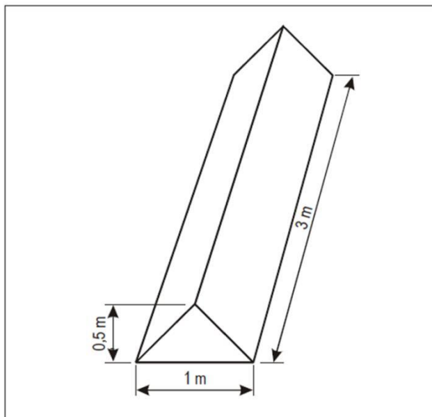
Figura 9-1 Balizas delimitadoras
