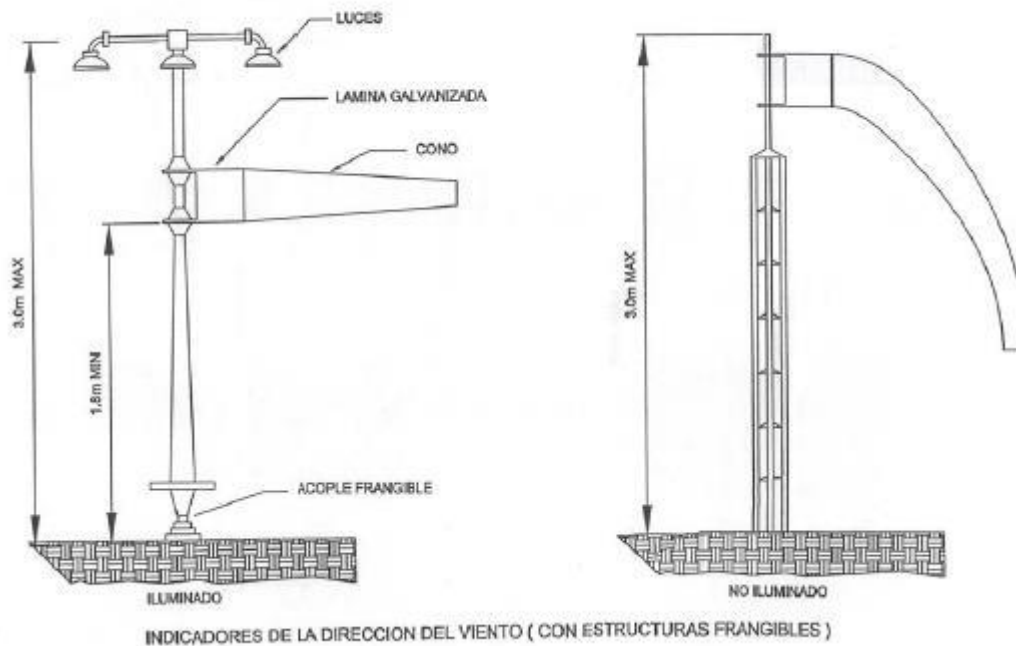
Figura 7-2. Estructuras frangibles
