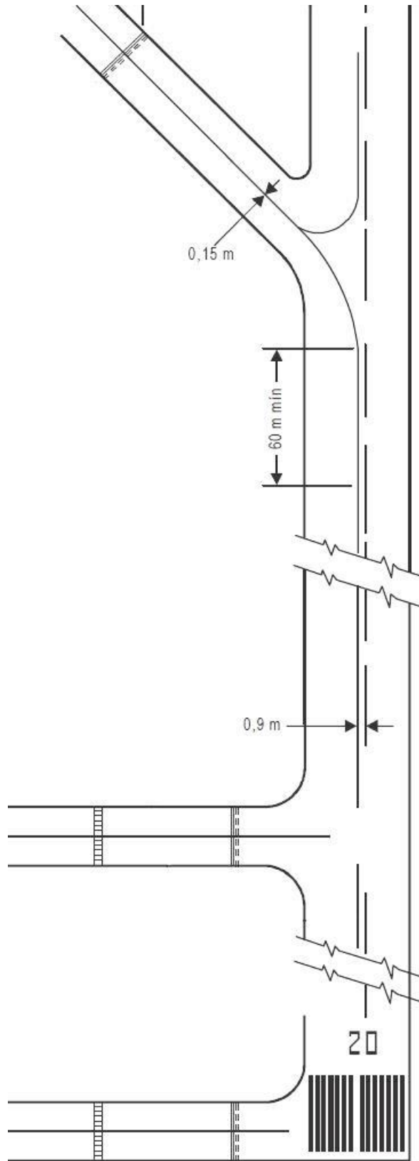
Figura 3-1-1. Señal de eje de calle de rodaje
