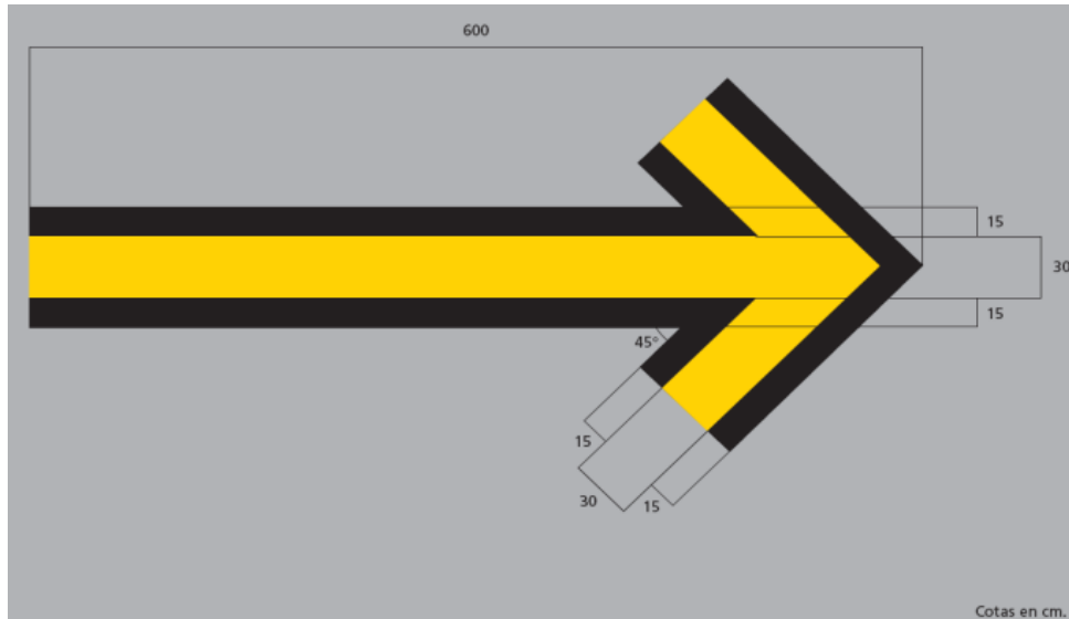
Figura 2-14-1. Señal de Barra de viraje
