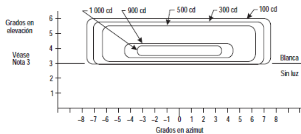
DIAGRAMA DE INDICACIÓN "DESCIENDA" DEL T-VASIS (DE NOCHE)
