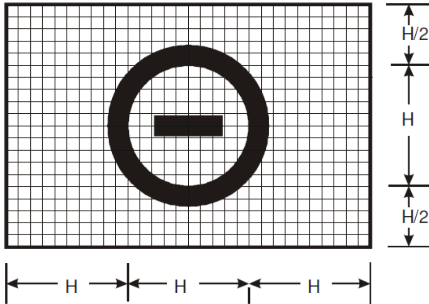
Figura ADJD-5. Ejemplo Letrero PROHIBIDA LA ENTRADA
