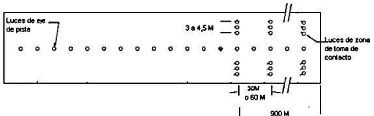
Figura 1-19-1. Luces de toma de contacto
