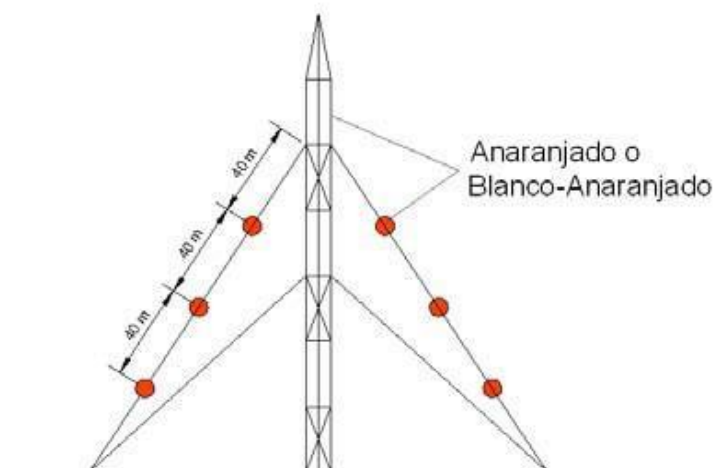
Figura 4-4. Señalamiento de las riendas para la erección de los mástiles de líneas de tensión
