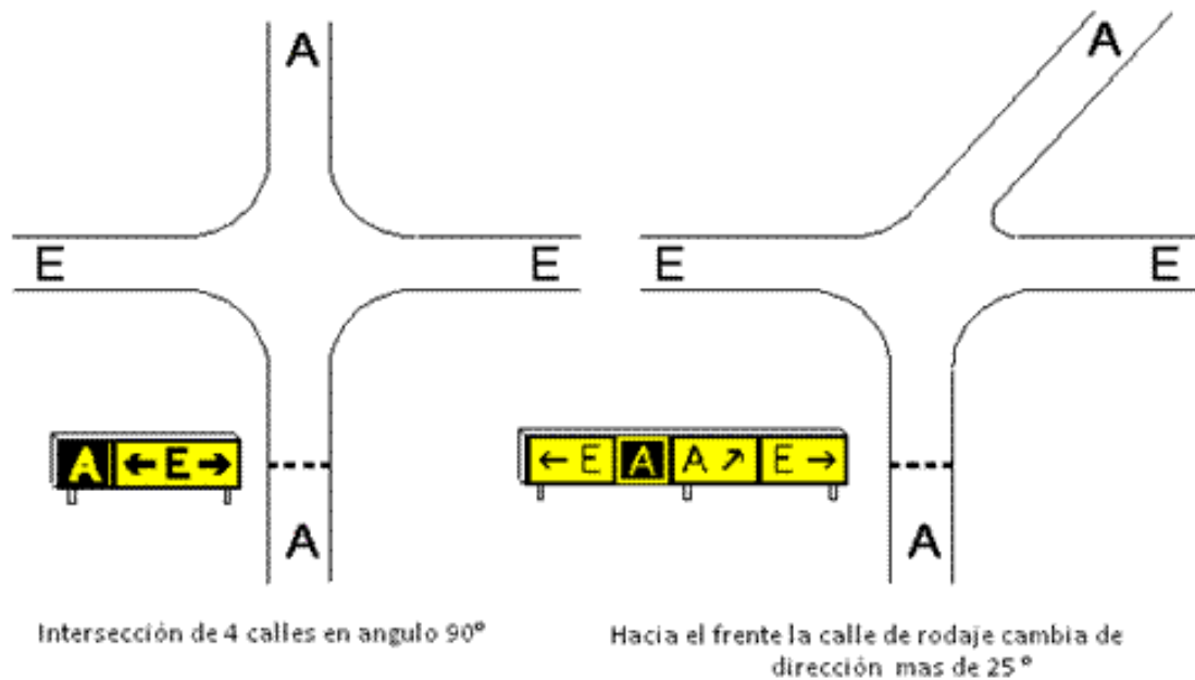
Figura 2-3-2. Caso B - Letreros de información
