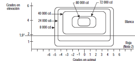
DIAGRAMA PARA LAS BARRAS DEL T-VASIS (DE DÍA)
