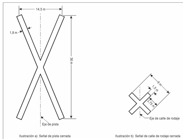
Figura 5-1-1. Señales de pista y de calle de rodaje cerradas
