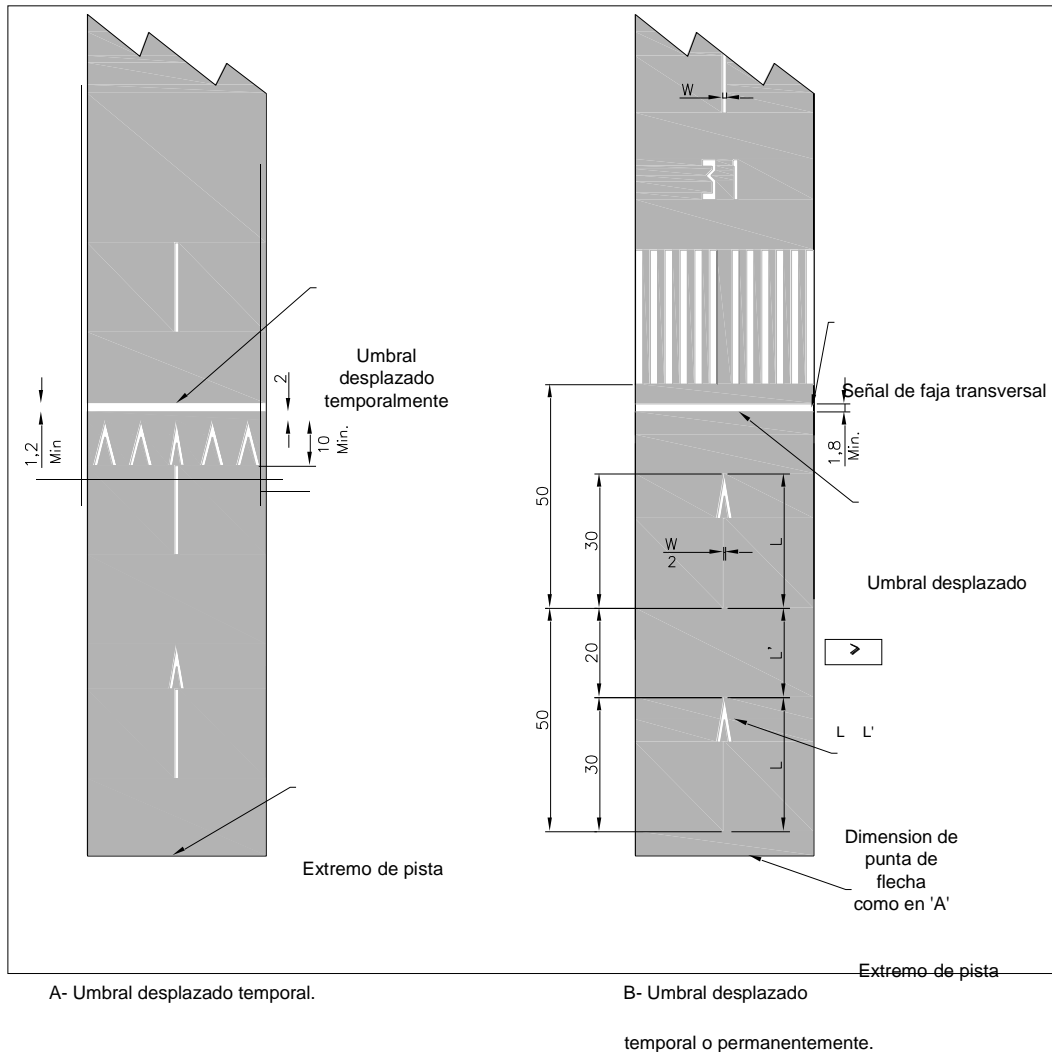
Figura 1-4-1. Señales de umbral desplazado
