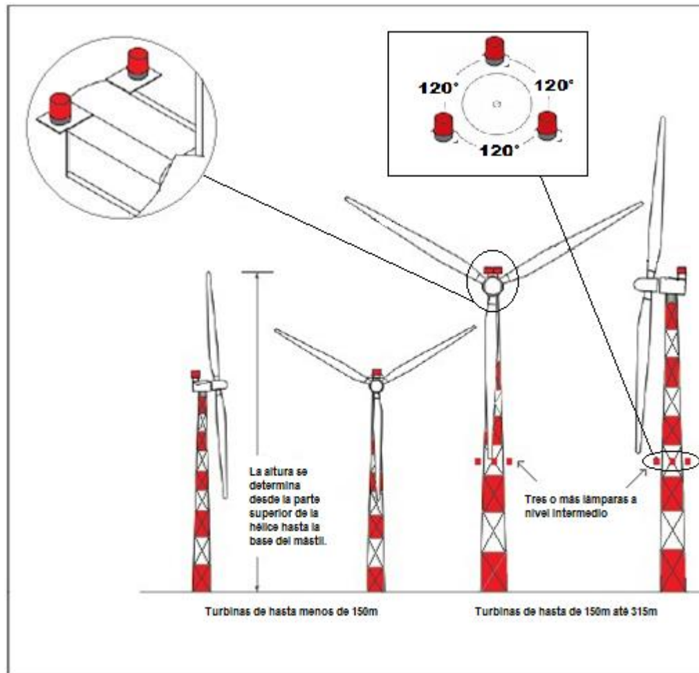
Figura 3-1-C: Señalamiento e iluminación de turbinas eólicas - condición en que os masts são construídos em estruturas treliçadas.
