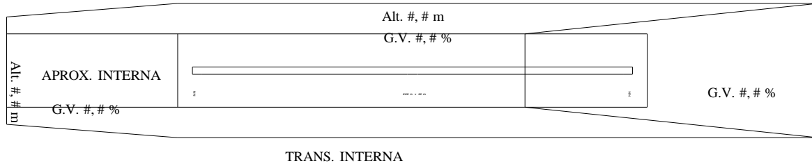
Figura 6-16 - Superficie de Aproximación Interna, Transición Interna y Aterrizaje Interrumpido
