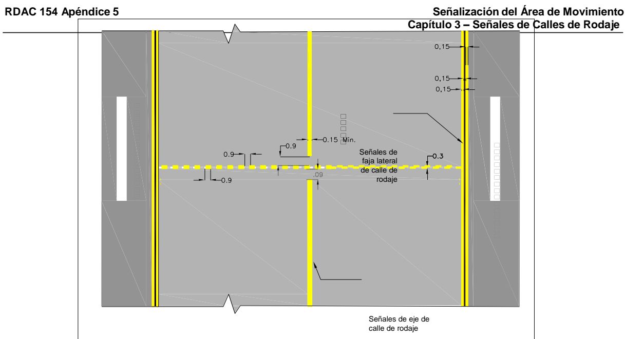
Figura 3-6-2. Señal de punto de espera intermedio.
