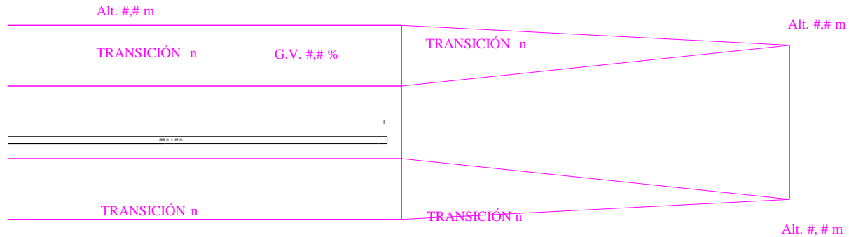
Figura 6-13 - Superficie de Transición
