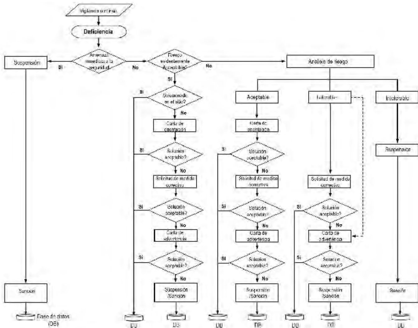
Figura 3-1 – Flujo del proceso de toma de decisiones y seguimiento de las deficiencias
