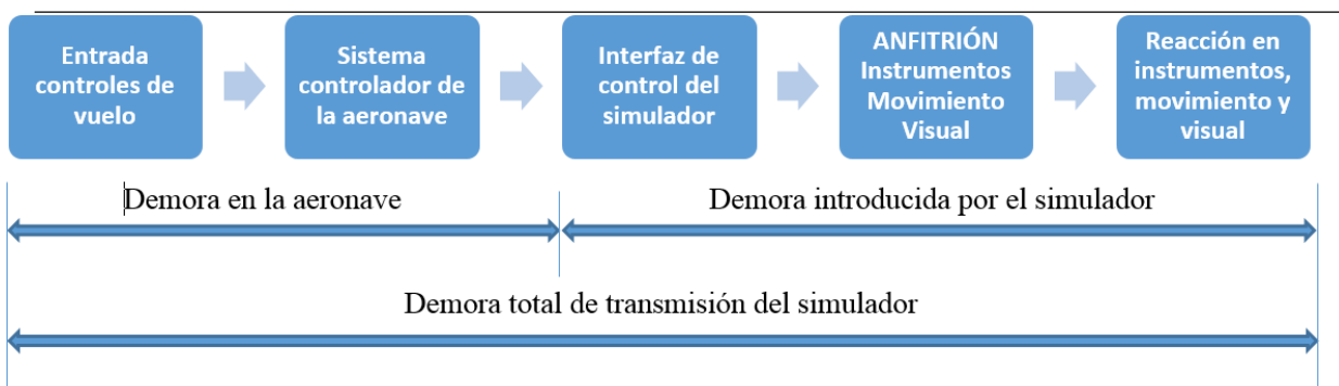
Figura 3.2G Tiempos de transmisión para simulación de aeronaves controladas por computador usando emulación de software de cajas negras de helicóptero
