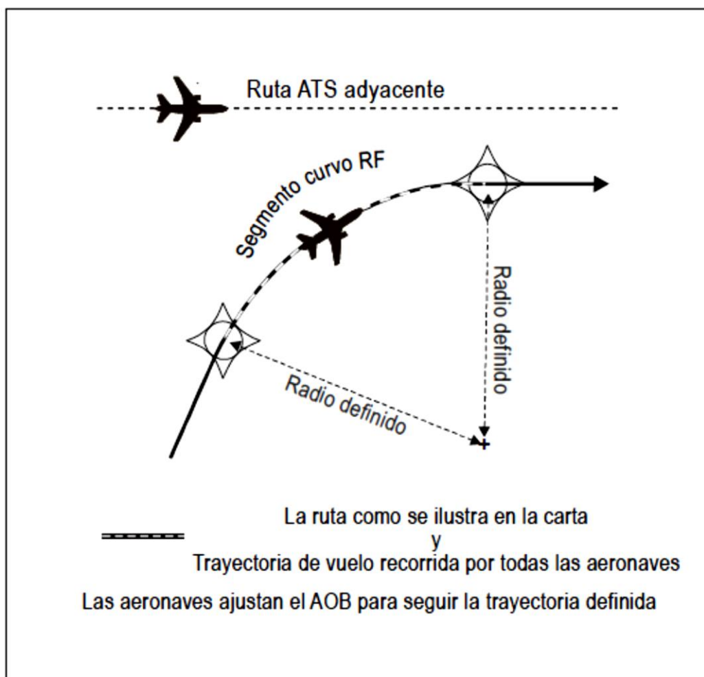
Arco de radio constante hasta un punto de referencia (RF)
