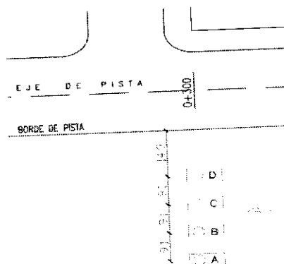
Figura Nro.1 Típica barra de ala del sistema PAPI.
