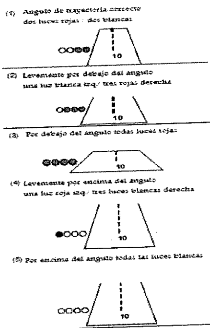
Figura Nro.2 Angulo de trayectoria de Barras de ala sistema PAPI.
