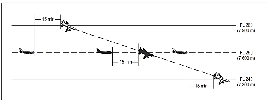
Figura 5-19B. Separación de 15 minutos entre aeronaves que descienden y por derrotas que se cruzan [véase 5.4.2.2.2.2 a)]
