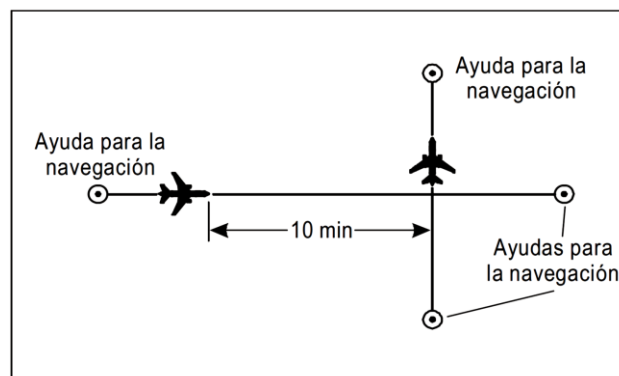
Figura 5-15. Separación de 10 minutos entre aeronaves por derrota que se cruzan y al mismo nivel [véase 5.4.2.2.1.2 b)]
