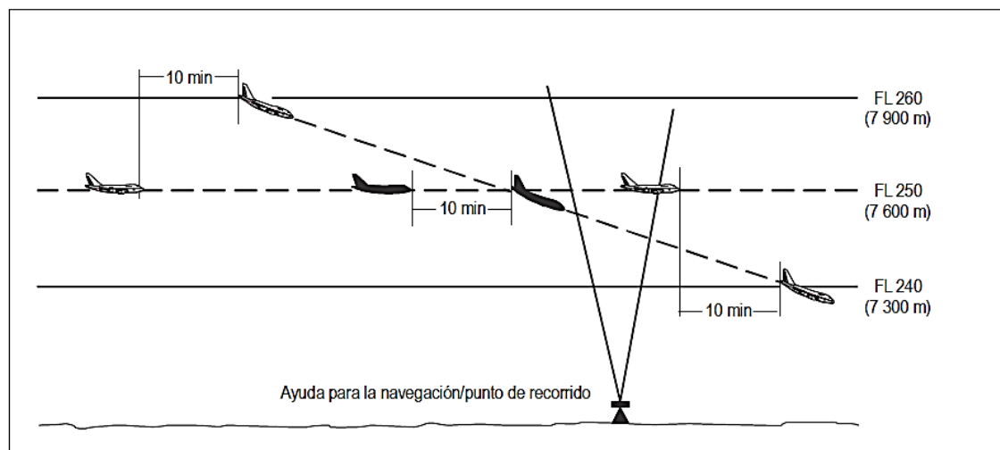
Figura 5-17B. Separación de 10 minutos entre aeronaves que descienden y por la misma derrota [véase 5.4.2.2.1 b)]
