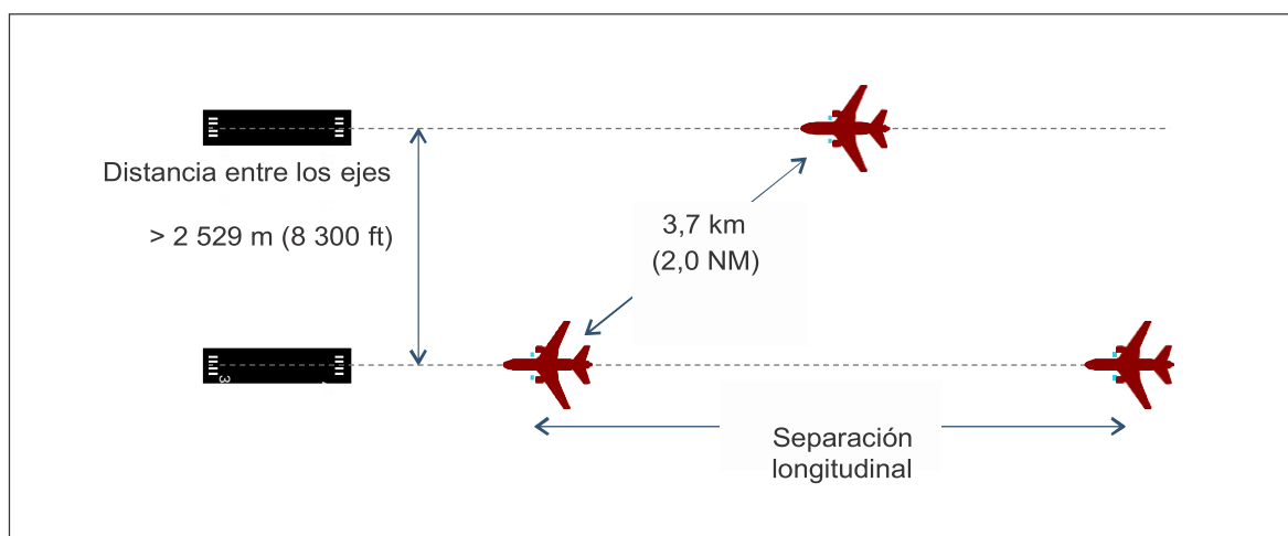
Figura 6-3. Separación diagonal para una distancia entre ejes mayor que 2 529 m (8 300 ft)
