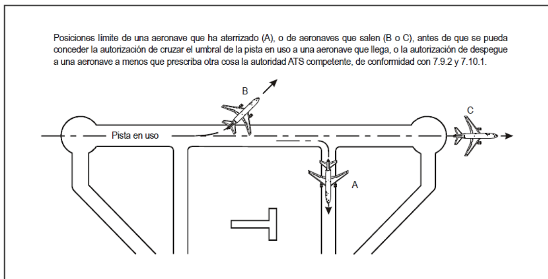
Figura 7-2. Separación entre aeronaves que llegan y salen (véanse 7.9.2 y 7.10.1)
