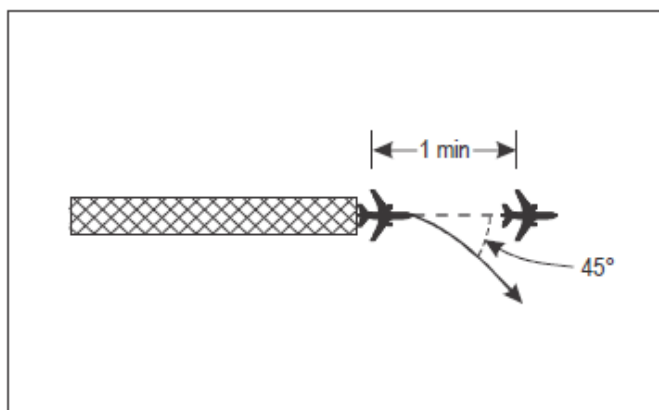
Figura 5-37. Separación de un minuto entre aeronaves que salen y siguen derrota divergentes por lo menos en 45° (véase 5.6.1)
