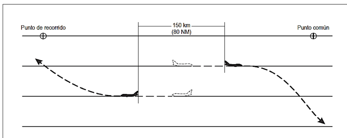
Figura 5-28. Separación de 150 km (80 NM) basada en RNAV entre aeronaves por derrotras opuestas (véase 5.4.2.5.7)
