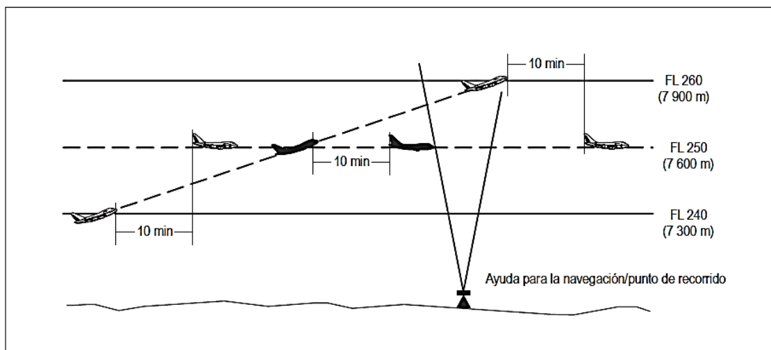
Figura 5-17A. Separación de 10 minutos entre aeronaves que ascienden y por la misma derrota [véase 5.4.2.2.1 b)]
