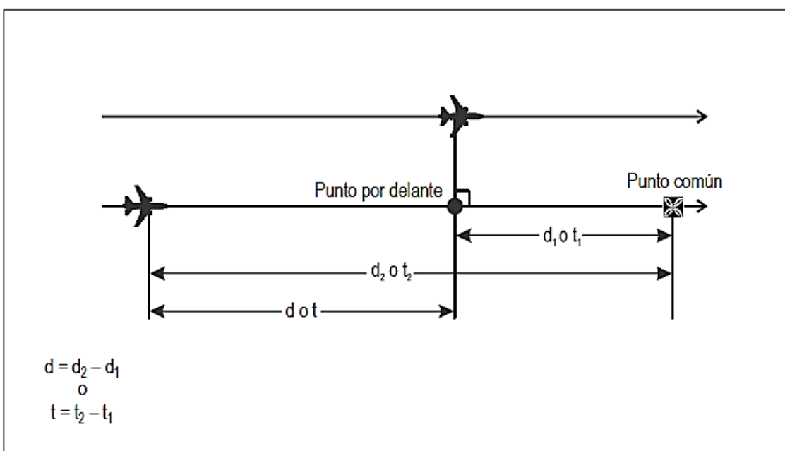
Figura 5-35. Cálculo de la distancia/tiempo longitudinal entre aeronaves — derrotas paralelas [véase 5.4.2.9.5 c)]
