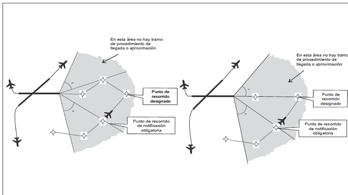
Figura 5-41. Área de protección de llegada
