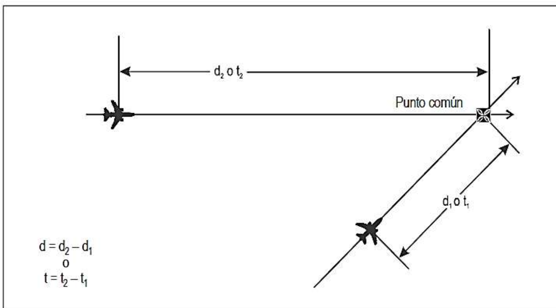
Figura 5-32. Cálculo de la distancia/tiempo longitudinal entre aeronaves — misma derrota, pero no idéntica y derrotas que se cruzan [véase 5.4.2.9.5 b)]
