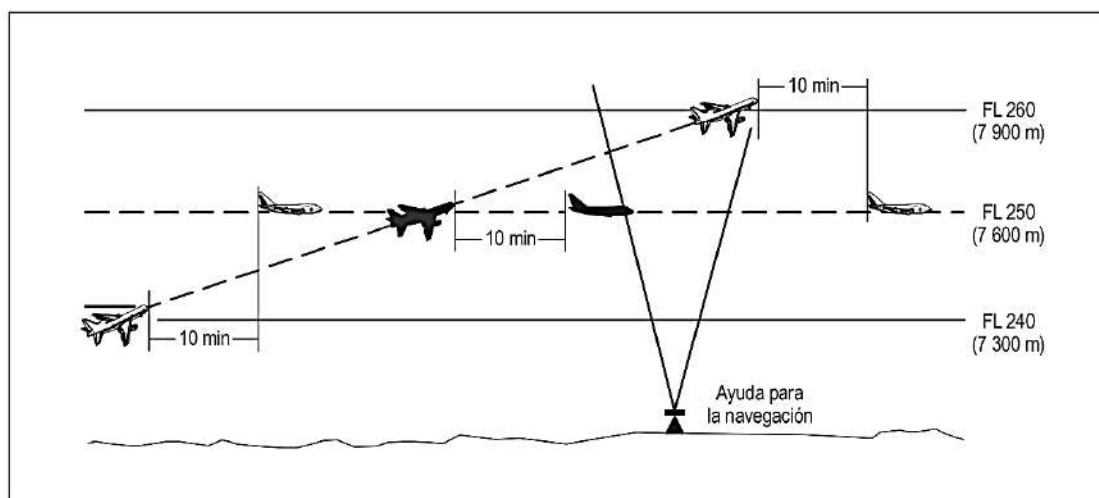
Figura 5-20A. Separación de 10 minutos entre aeronaves que ascienden y por derroteros que se cruzan [véase 5.4.2.2.2.2 b)]
