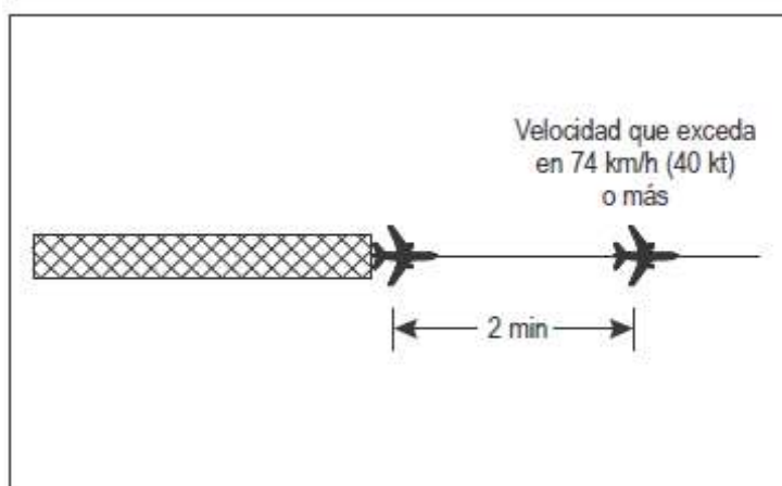
Figura 5-38. Separación de dos minutos entre aeronaves que siguen la misma derrota (véase 5.6.2)
