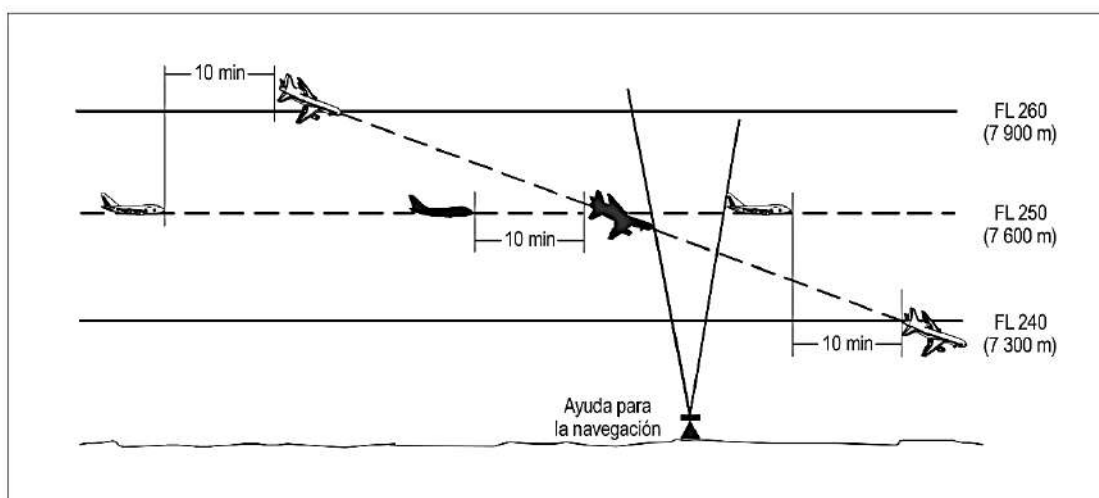
Figura 5-20B. Separación de 10 minutos entre aeronaves que descienden y por derroteros que se cruzan [véase 5.4.2.2.2.2 b)]
