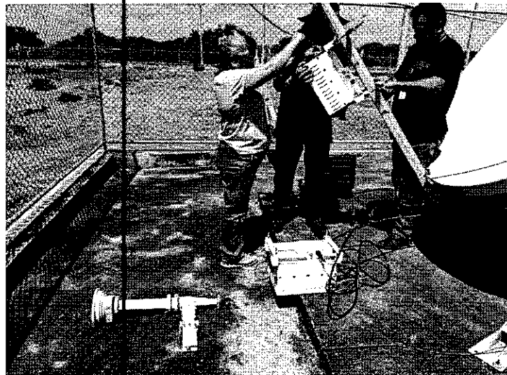
CAMBIO DE BUC Y DE FEED HORN
