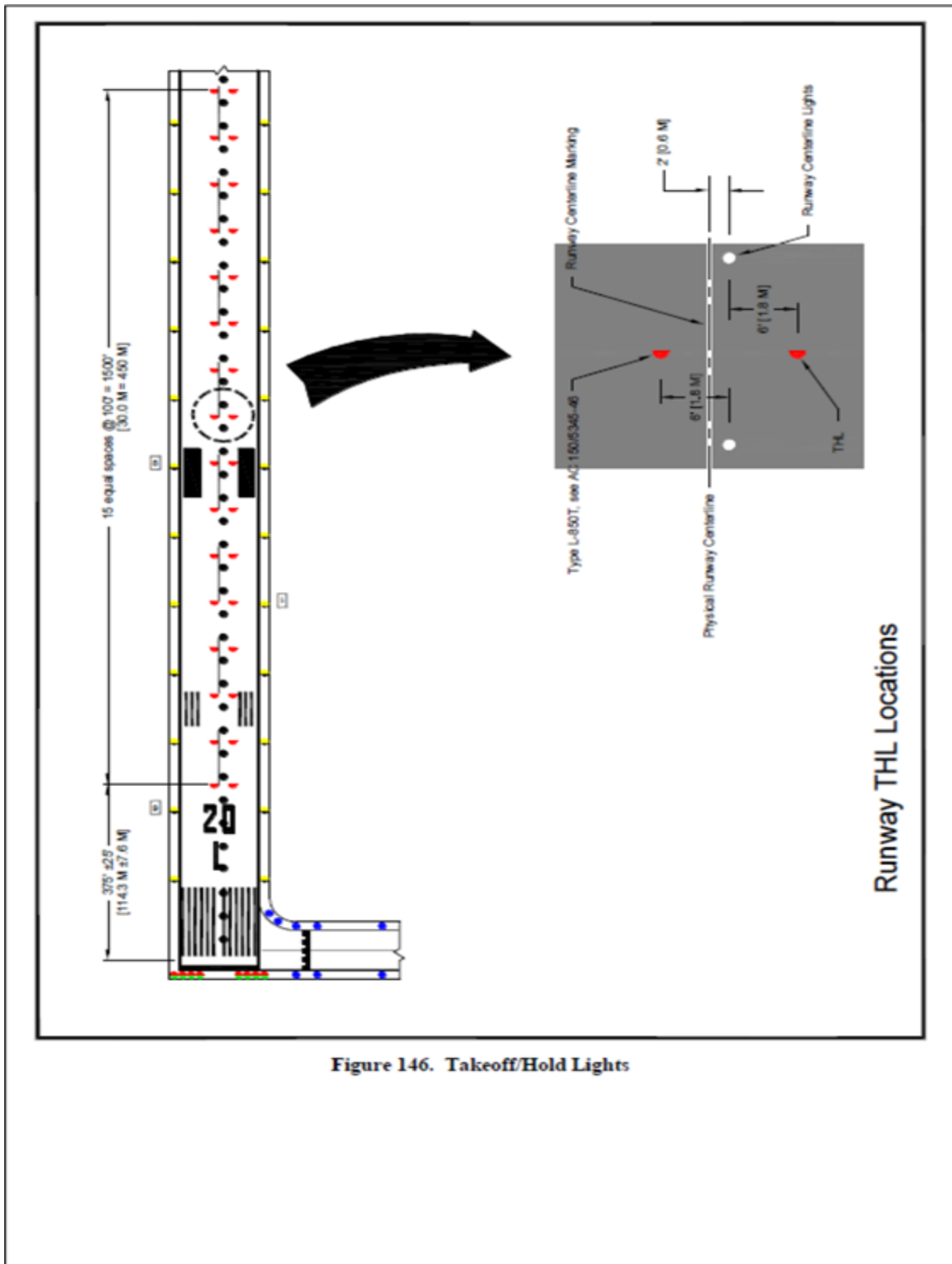
Figura 1-41-4 Sistema THL
