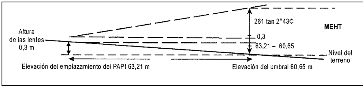
Figura 1-10-7. Datos de levantamiento topográfico y corrección de la posición nominal del PAPI con IL
