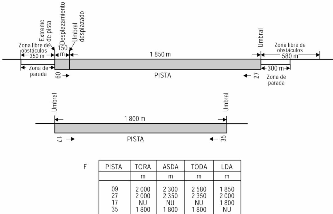
Figura 1-6-2. Determinación de las Distancias Declaradas.
