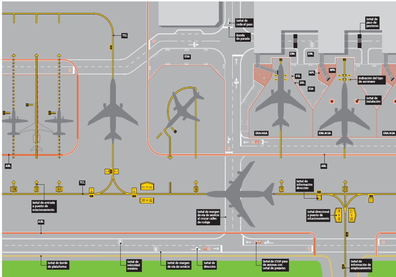
Figura 2-17-2. Vista general de señales
