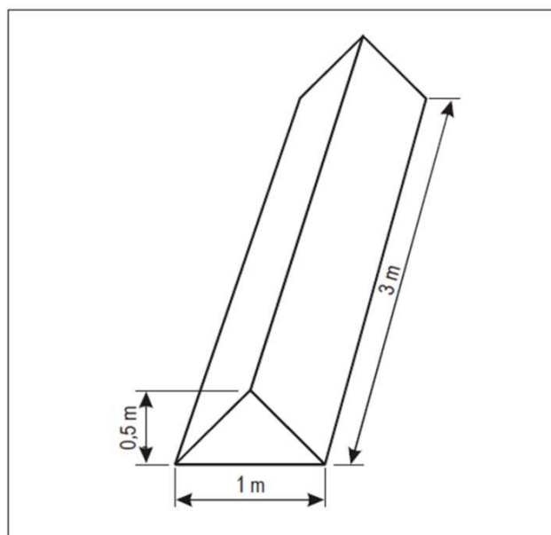
Figura 9-1 Balizas delimitadoras
