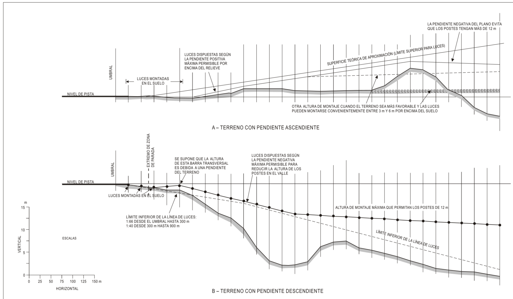
Figura ADJF-4. Tolerancias verticales de instalación
