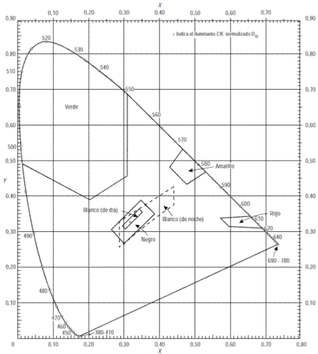
Figura ADJA-3-3. Colores de los letreos y paneles trans iluminados (iluminación interna) o luminiscentes
