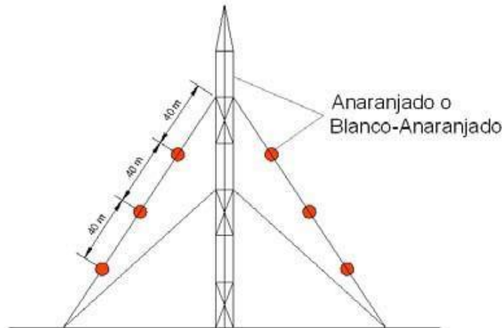
Figura 4-4. Señalamiento de las riendas para la erección de los mástiles de líneas de tensión con esferas de colores
