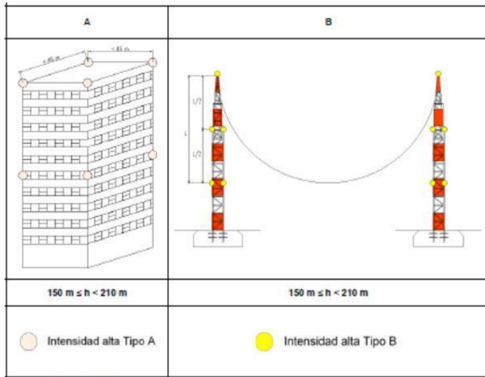
Figura 2-3-10 Ejemplo de Luces de obstáculos de alta intensidad A y B ALTURA ( 150 m \leq H < 210 m )
