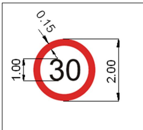
Figura 4-1-4 Detalle de señales límite de velocidad
