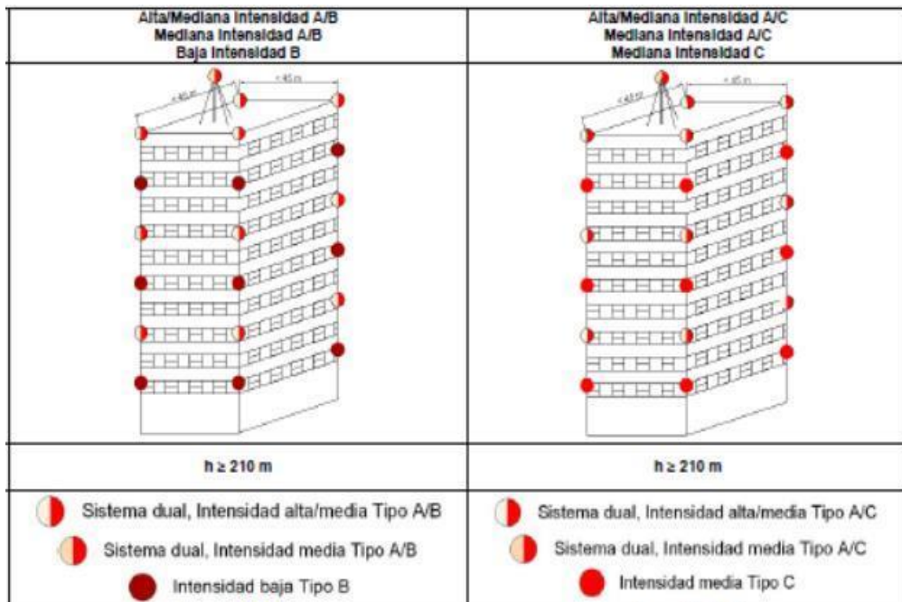
Figura 2-3-11 Ejemplo de Luces de obstáculos de alta y media intensidad A y B/ A y C
