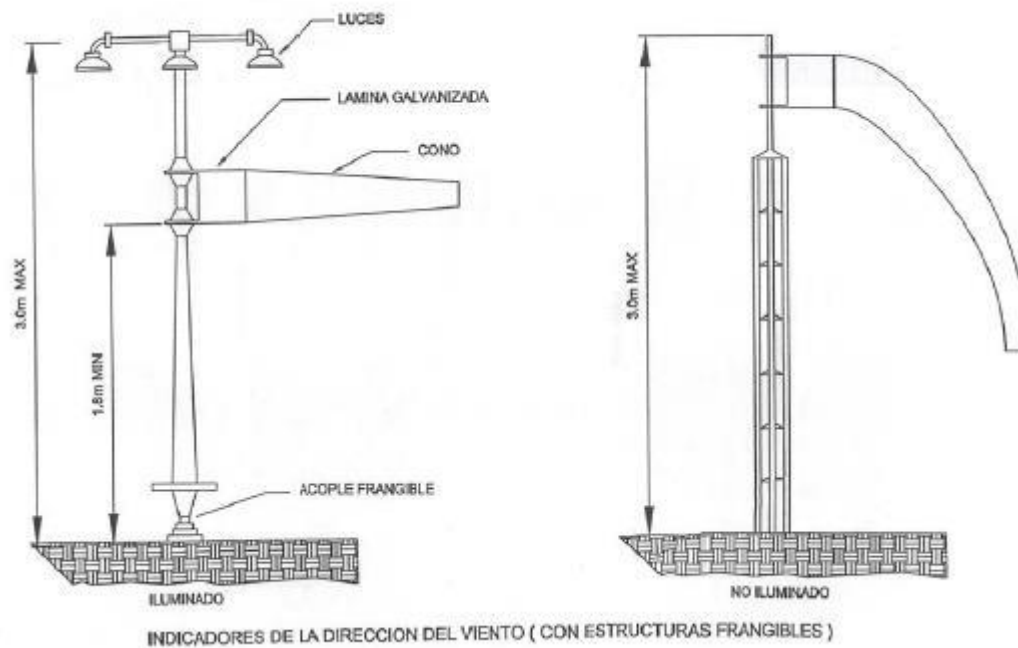
Figura 7-2. Estructuras frangibles
