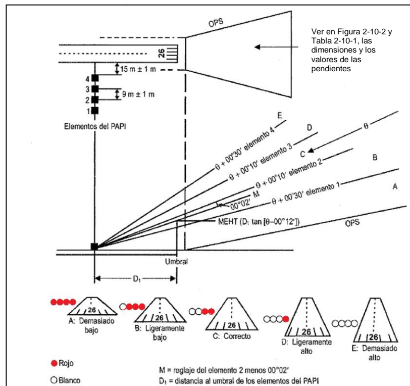
Figura 1-10-4. Disposición de los elementos del PAPI
