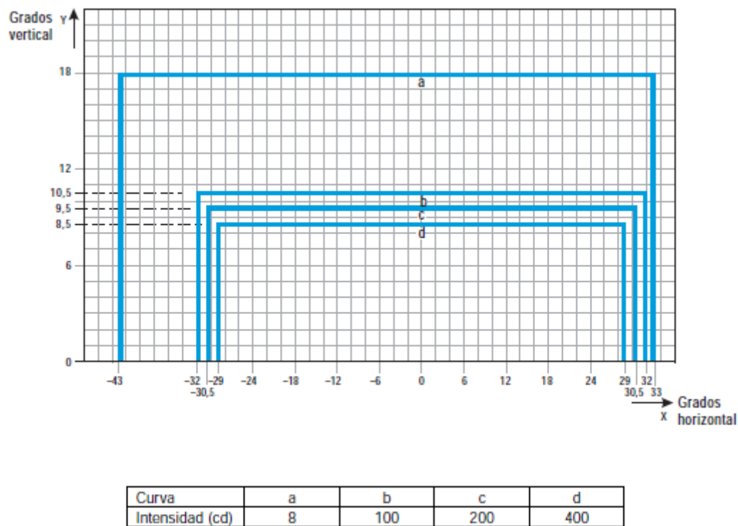
Figura A2-19. Diagrama de isocandelas para las luces de eje de calle de rodaje (con espaciado de 7,5 m), de barra de prohibición de acceso y de barra de parada de alta intensidad en tramos curvos, previstas para ser utilizadas en un sistema avanzado de guía y control del movimiento en la superficie, en el que se requieran intensidades luminosas más elevadas
