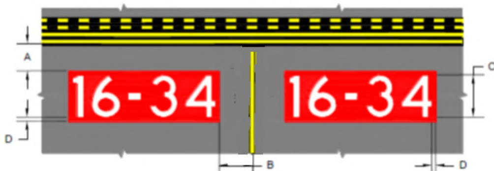
Figura 4-2-3. Dimensiones Señal con instrucciones obligatorias
