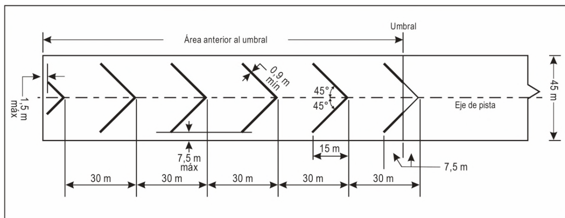
Figura 5-3-1. Señal anterior al umbral
