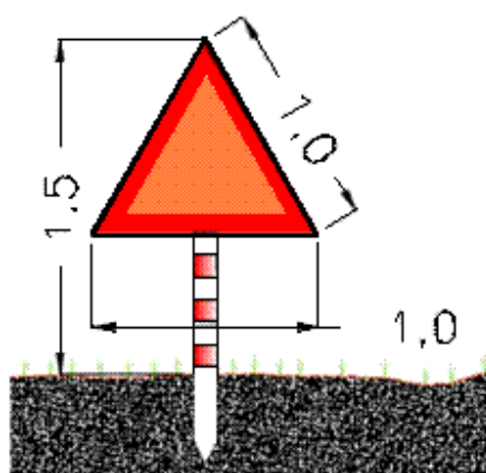
Figura 6-9-1 Detalle de las balizas de final de pistas no pavimentadas
