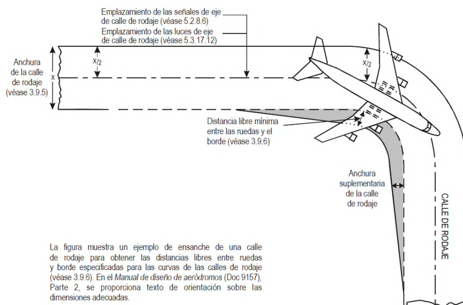
Figura 1-19-2 Curva de calle de rodaje
