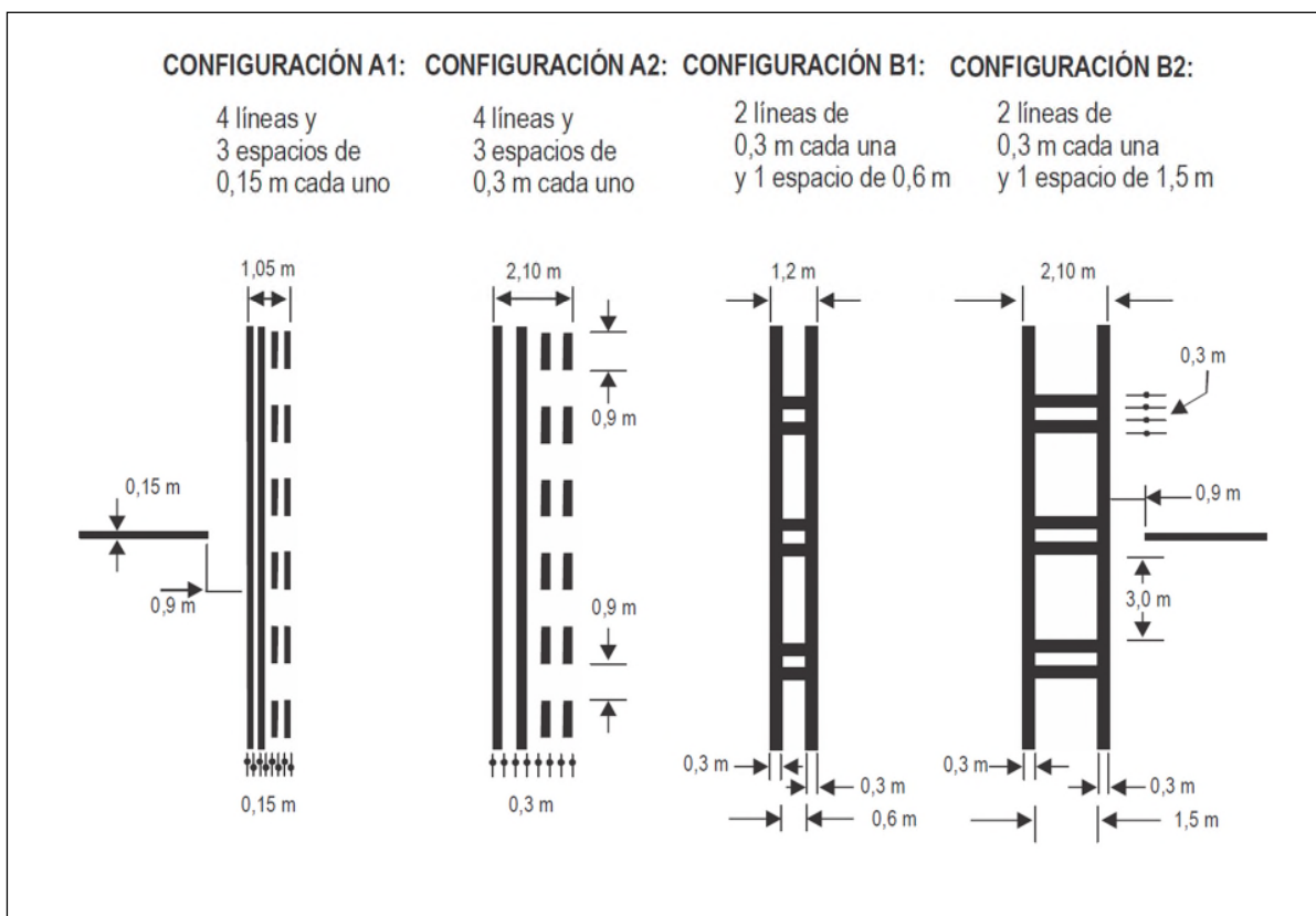
Figura 3-5-2 Señales del punto de espera de la pista
