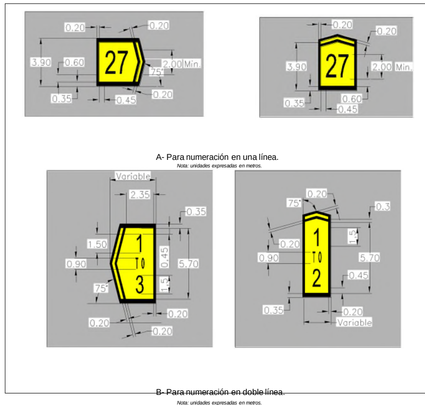
Figura 2-9-1. Señal direccional a puestos de estacionamiento de aeronaves
