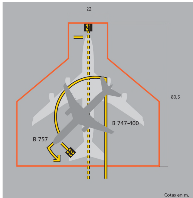
Figura 2-25-6. Estacionamientos superpuestos para distintos tipos de aeronaves.
