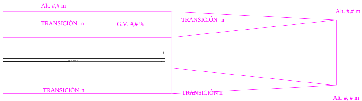
Figura 6-13 - Superficie de Transición
