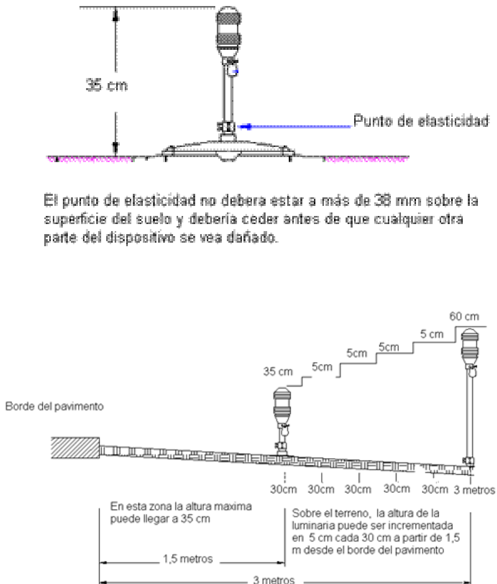
Figura 1-1-1. Altura de las luces elevadas
