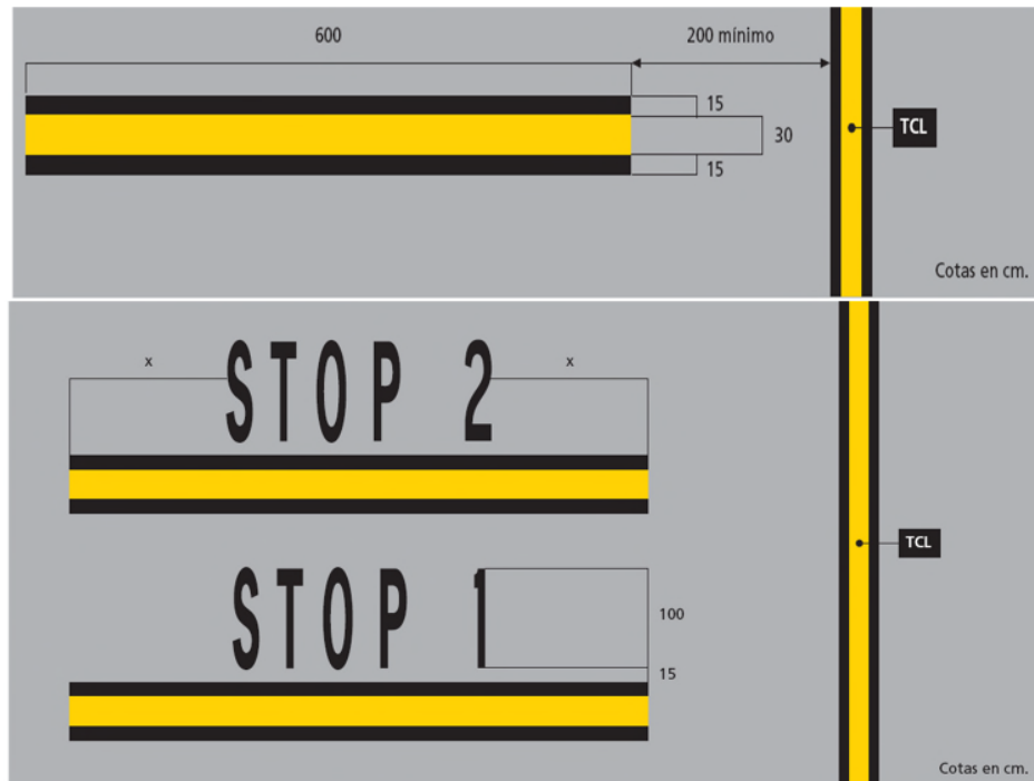
Figura 2-17-1. Señal de Barra de Parada
