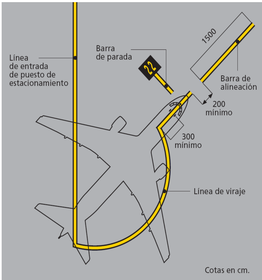
Figura 2-19-2. Señal de Barra de alineación
