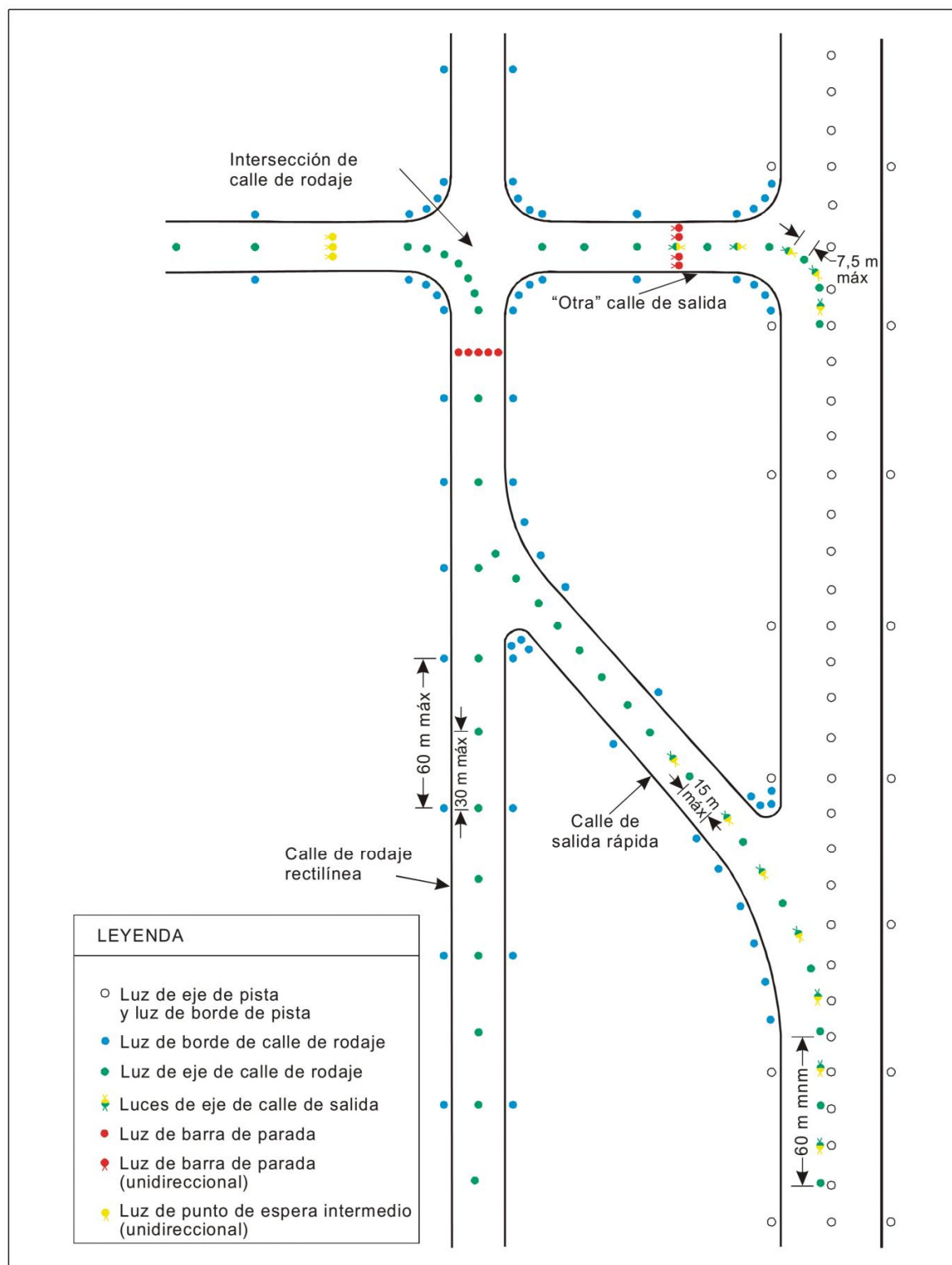
Figura 1-22-1. Iluminación de calles de rodaje
