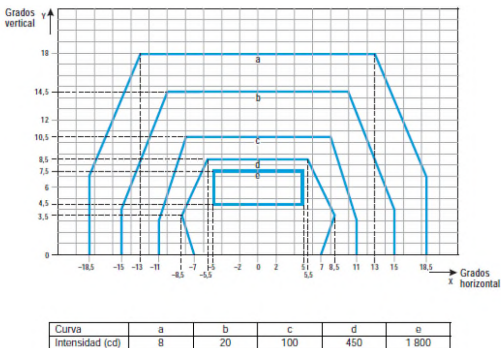
Figura ADJB-18. Diagrama de isocandelas para las luces de eje de calle de rodaje (con espaciado de 15 m), de barra de prohibición de acceso y de barra de parada de alta intensidad en tramos rectos, previstas para ser utilizadas en un sistema avanzado de guía y control del movimiento en la superficie, en el que se requieran intensidades luminosas más elevadas
