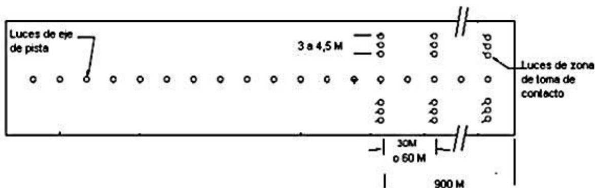
Figura 1-19-1. Luces de toma de contacto
