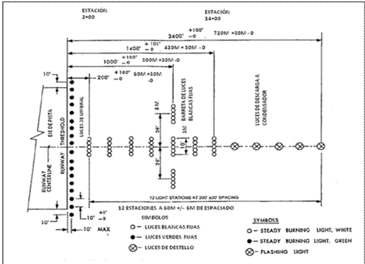
Figura ADJJ2. Configuración MALSR medidas en pies/metros
