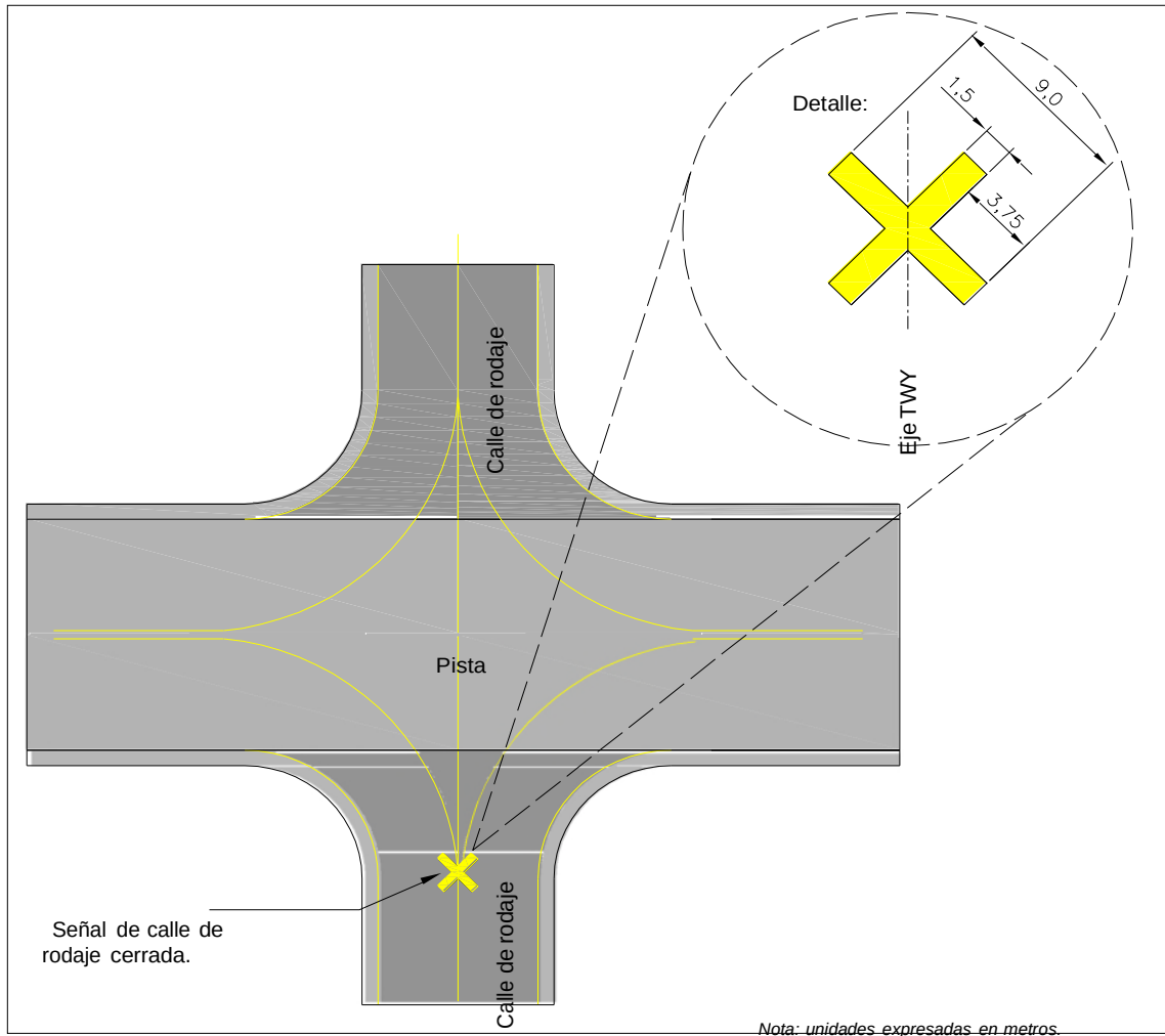
Figura 5-1-2 Señales de calle de rodaje cerradas – emplazamiento respecto a una pista en uso
