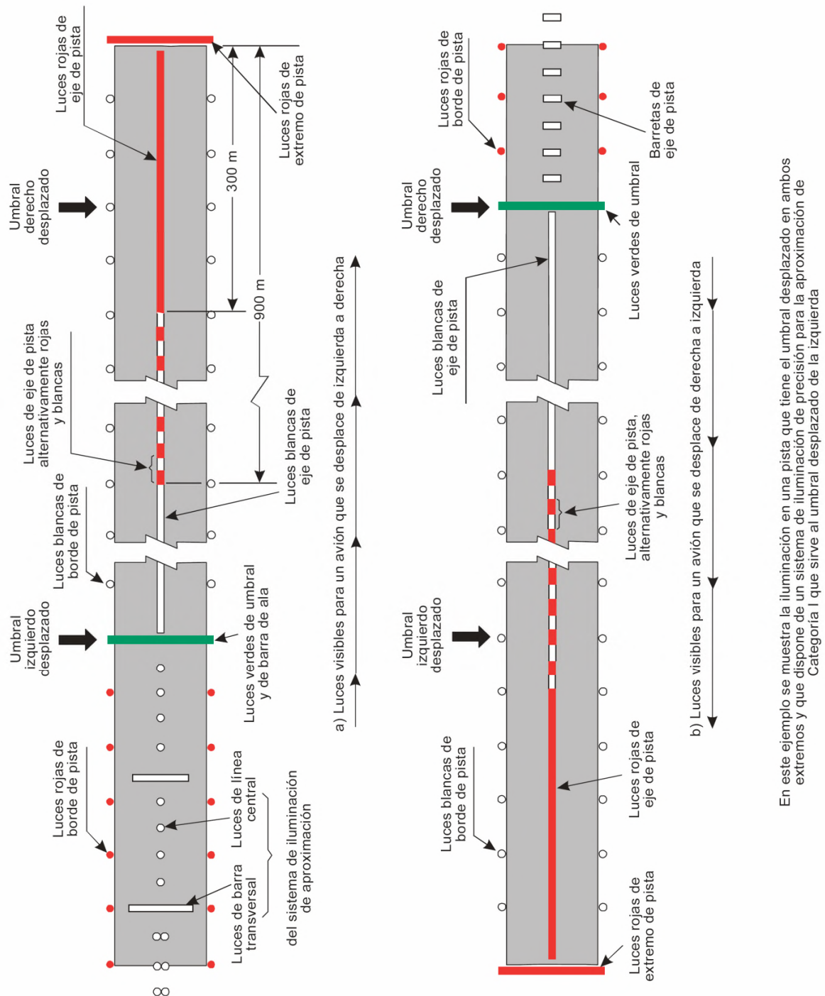
Figura 1-17-1. Ejemplo de iluminación de aproximación y de la pista en las pistas con umbrales desplazados
