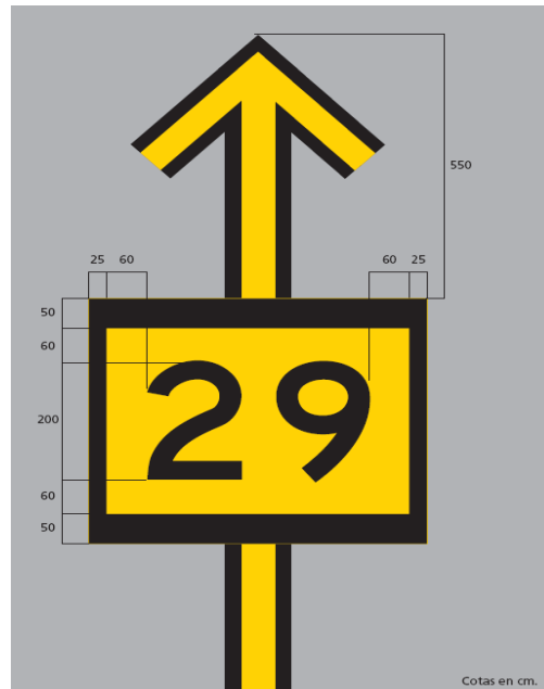
Figura 2-11-4. Identificación de puesto de estacionamiento con dos direcciones de rodajes hacia el puesto
