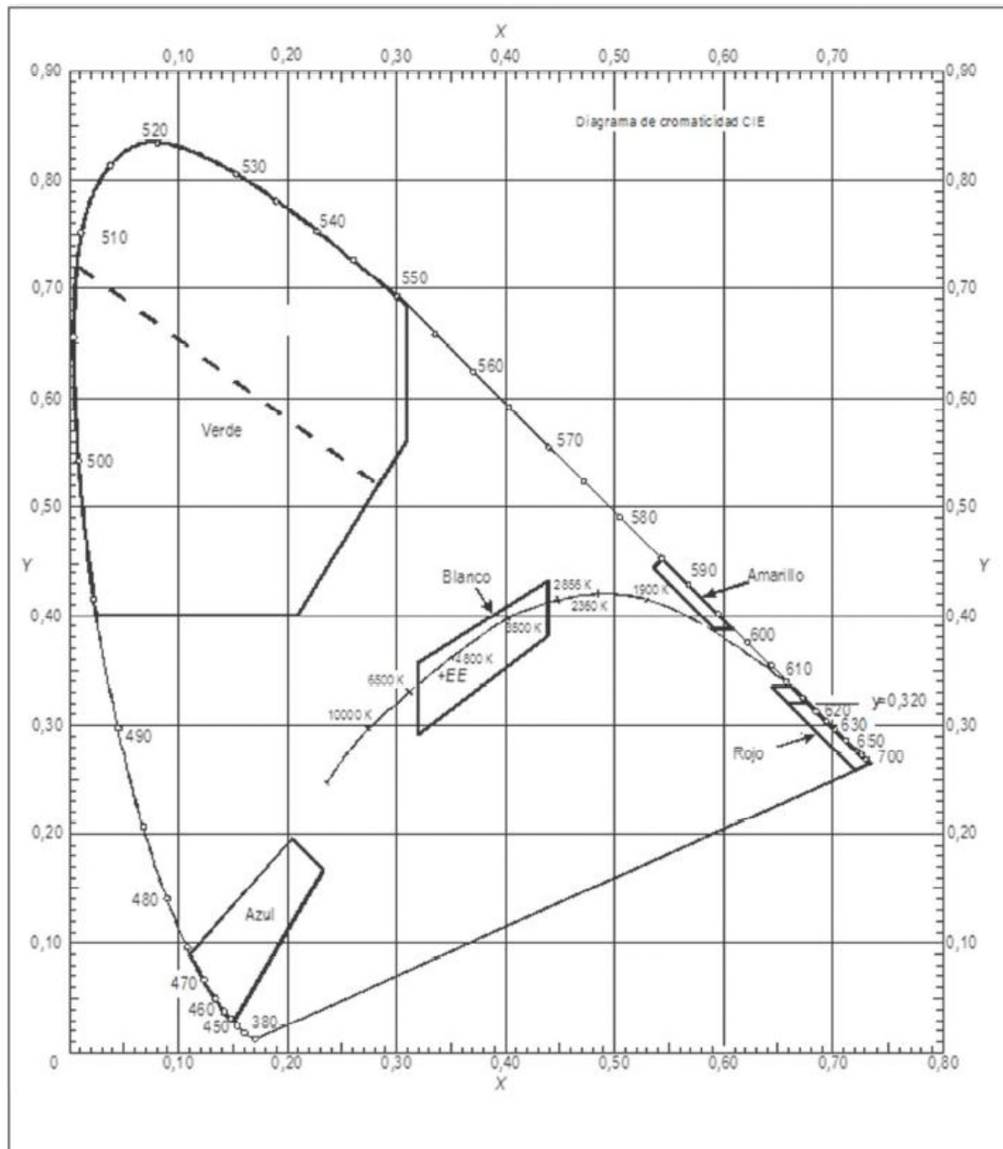
Figura ADJA-2-1b. Colores de luces aeronáuticas de superficies (lámparas de estado sólido)
