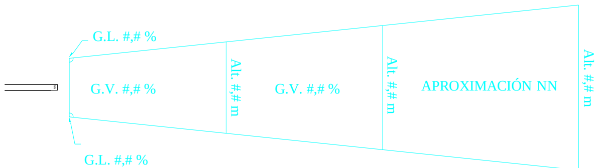
Figura 6-11 - Superficie de Aproximación
