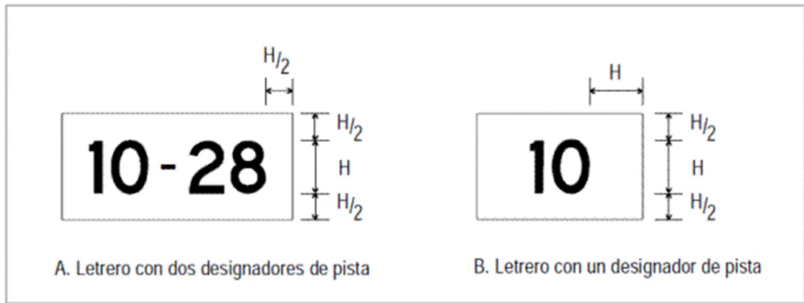
Figura ADJD-7. Dimensiones de los letreros
