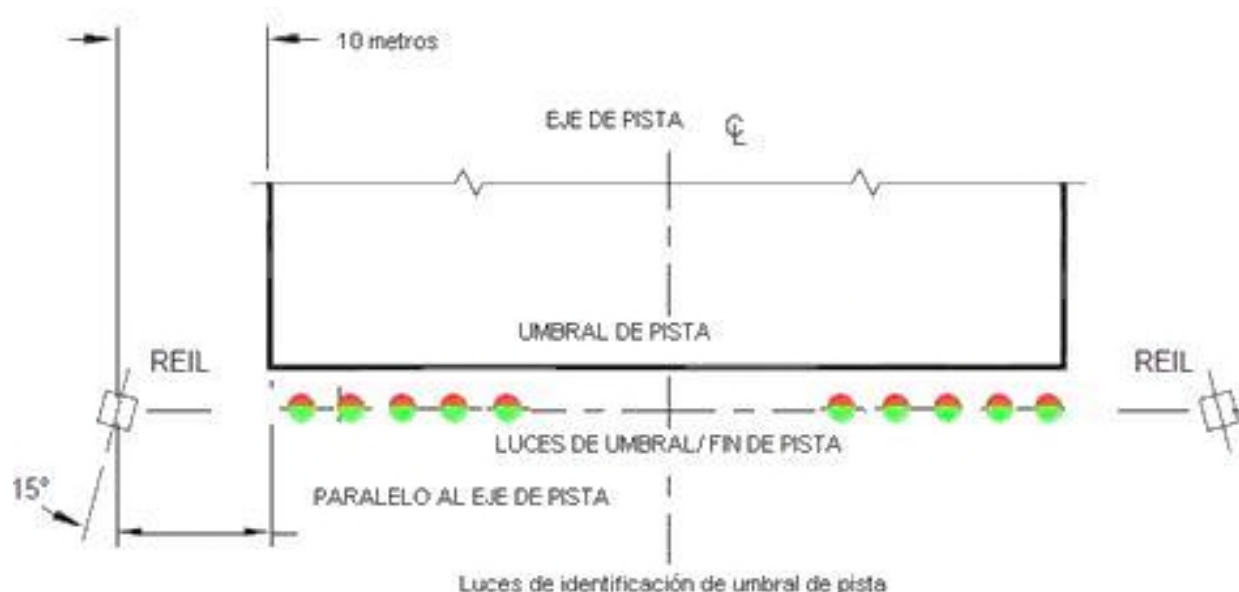
Figura 1-13-1. Luces de Identificación de umbral de pista
