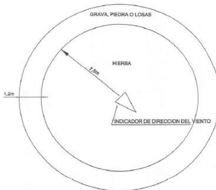
Figura 7-3. Detalle de la señalización del emplazamiento del indicador de la dirección del viento
