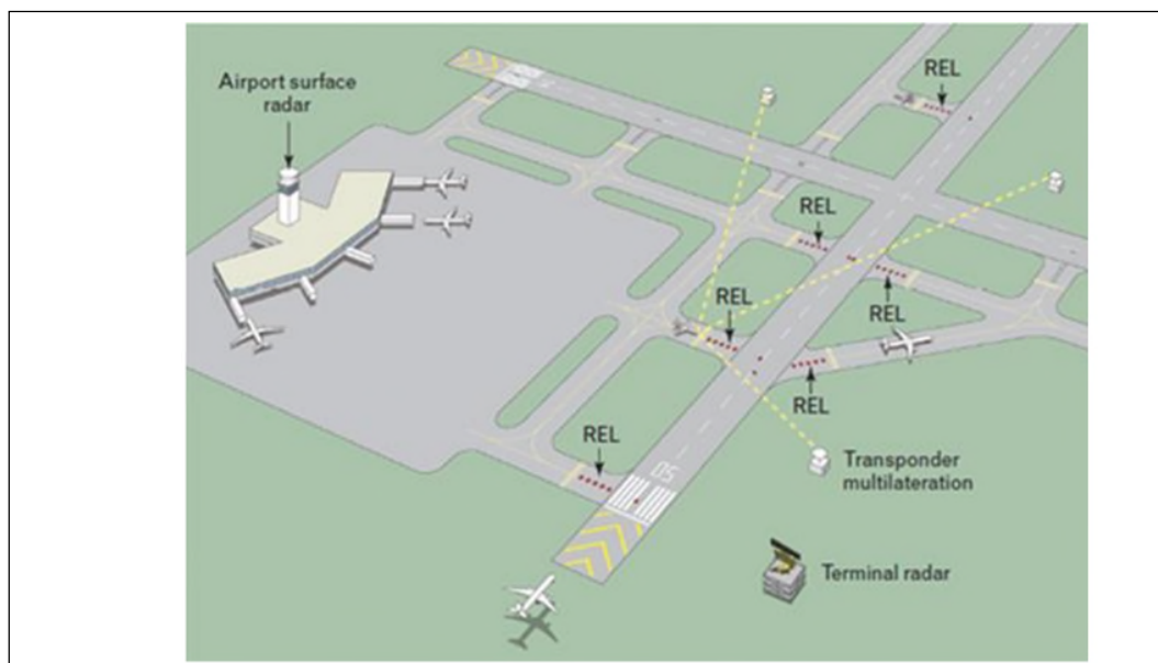
Figura 1-41-1 Sistema autónomo de advertencia de incursión en la pista (ARIWS) Emplazamiento
