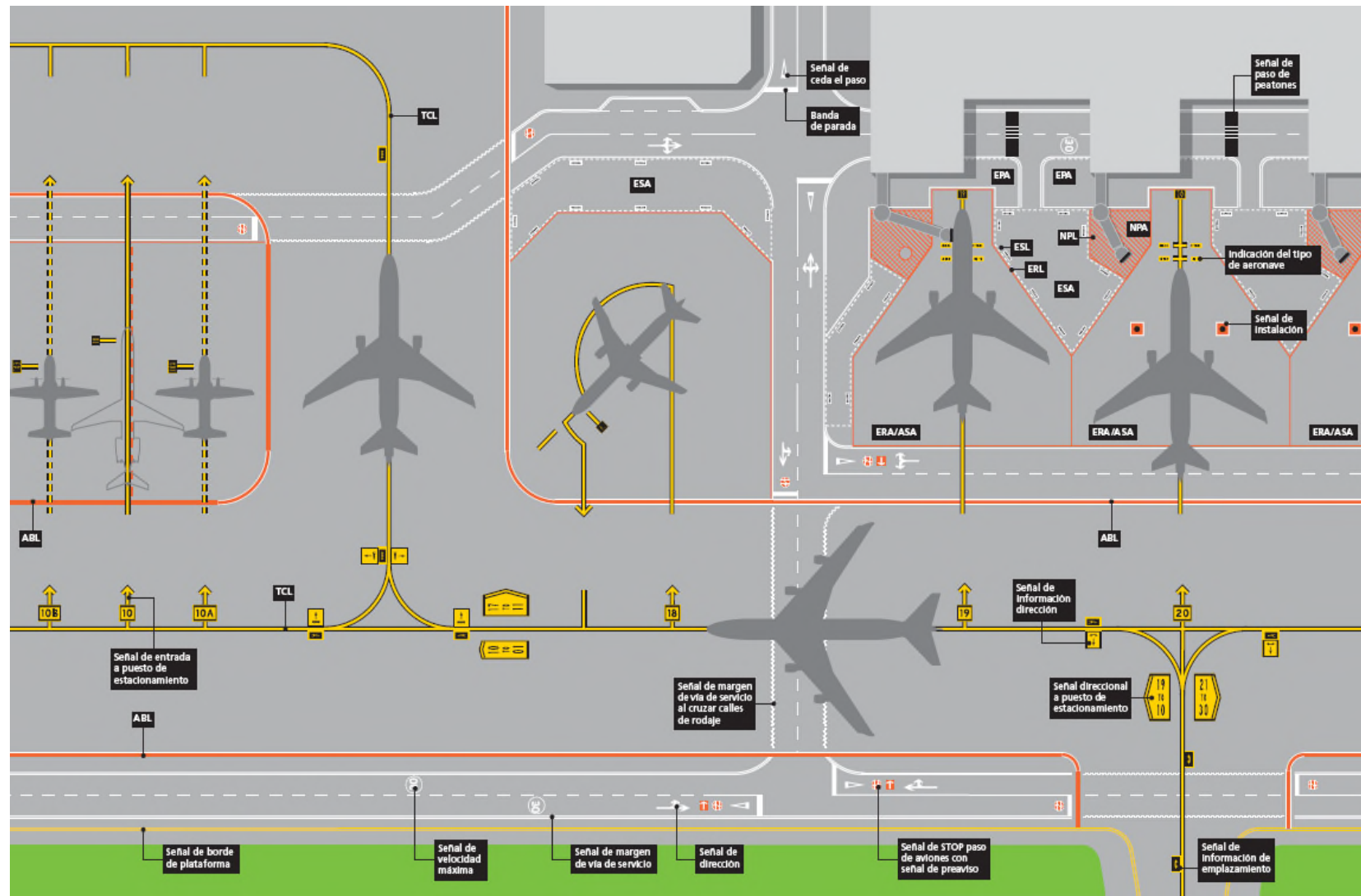
Figura 2-17-2. Vista general de señales
