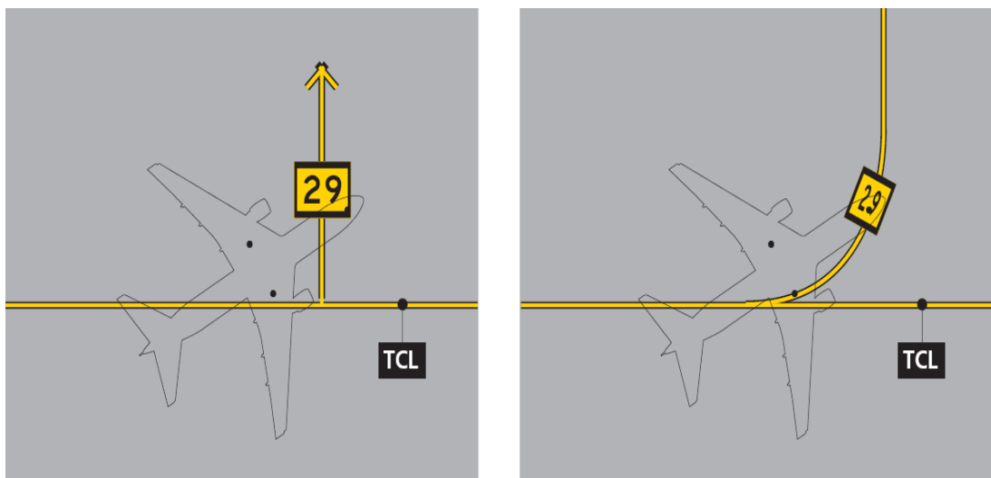
Figura 2-10-2. Señal de entrada a puestos de estacionamiento de aeronaves, recta y simple
