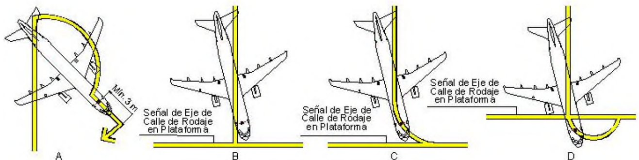
Figura 2-13-2. Señal de salida de puesto de estacionamiento, con giro, recta, simple y desplazada
