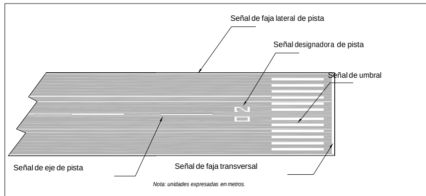
Figura 1-2-1. Señales de pista
