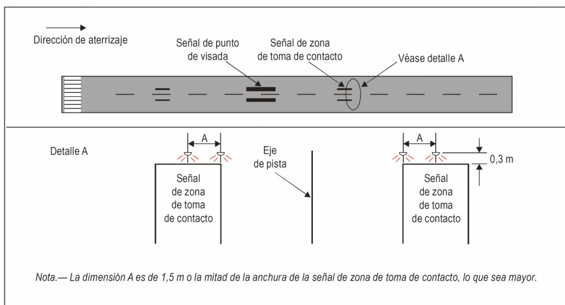
Figura 1-19-3 Luces simples de toma de contacto
