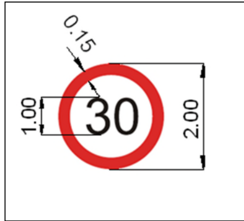
Figura 4-1-4 Detalle de señales límite de velocidad
