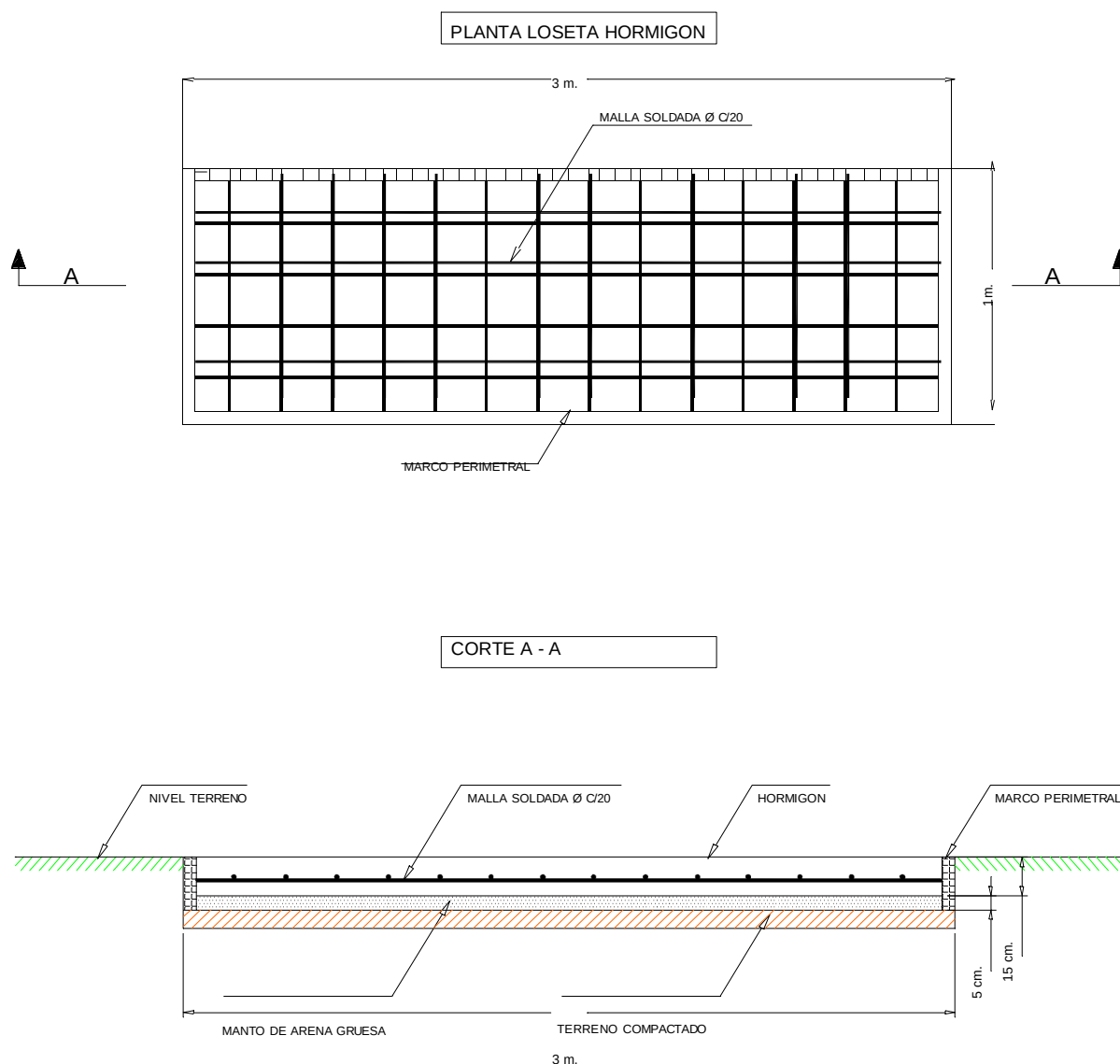
Figura 6-5-1. Características constructivas sugeridas para las señales de borde de pista no pavimentada
