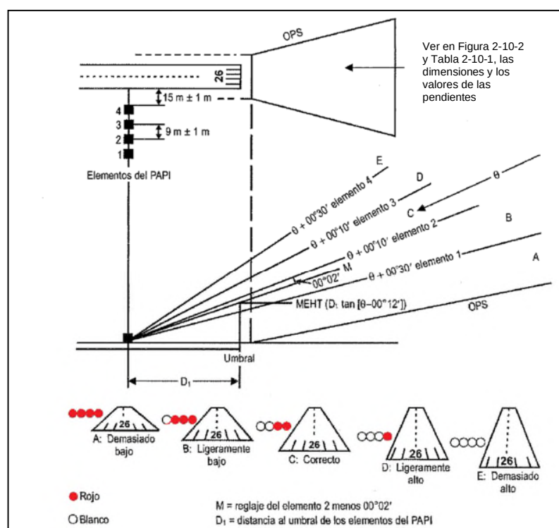
Figura 1-10-4. Disposición de los elementos del PAPI
