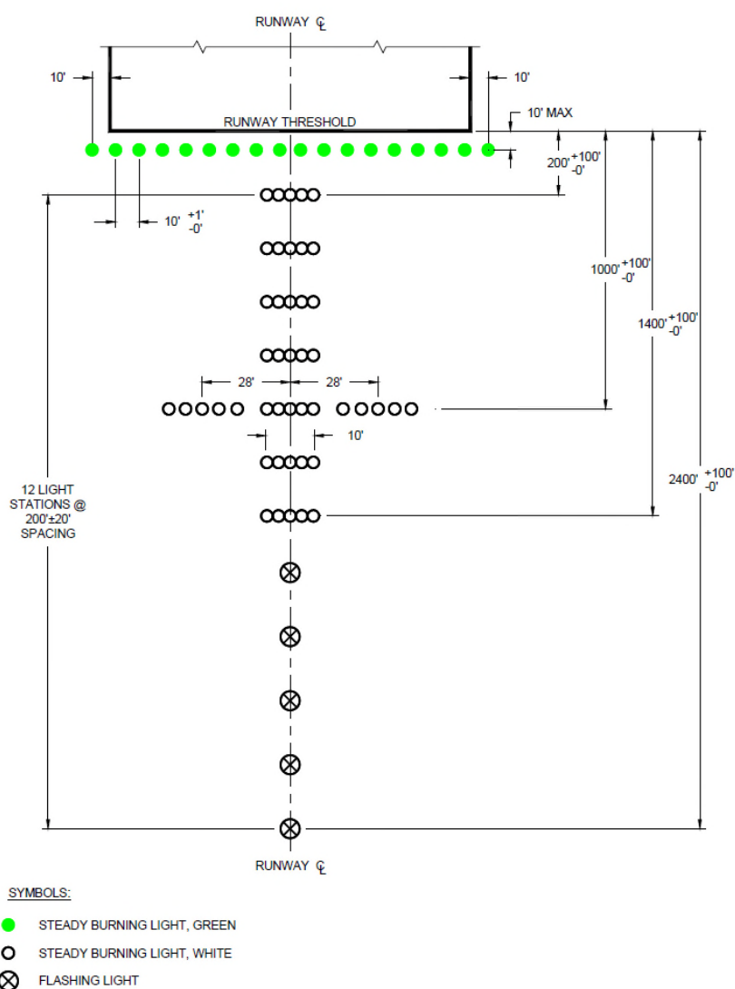
Figura ADJJ1. Configuración MALSR medidas en pies
