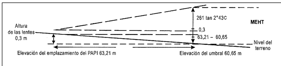
Figura 1-10-7. Datos de levantamiento topográfico y corrección de la posición nominal del PAPI con ILS
