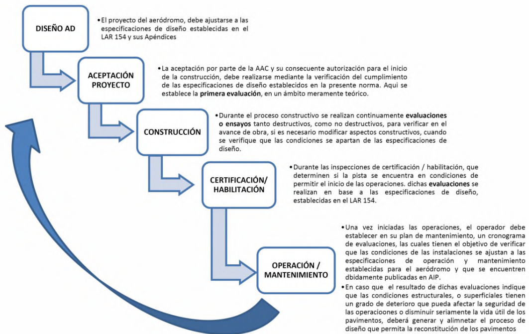
Figura 1-1. Diagrama de vida de un pavimento
