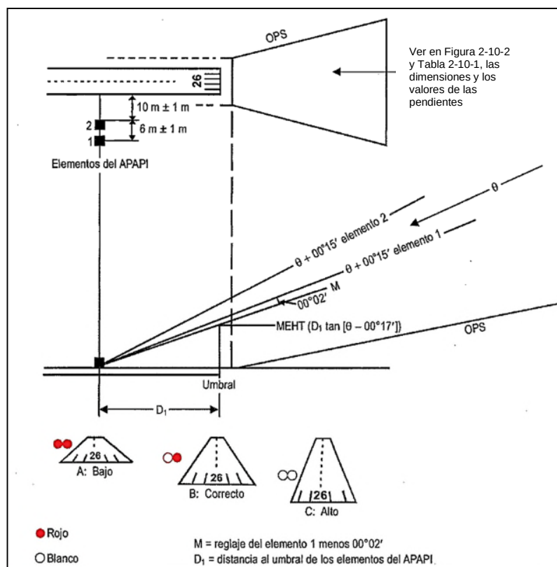
Figura 1-10-5. Disposición de los elementos del APAPI
