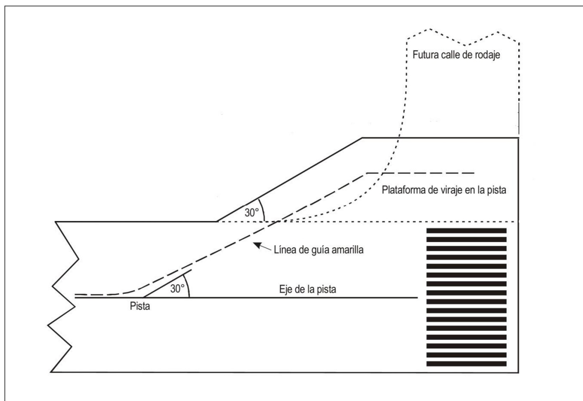
Figura 1-14-2. Detalle de Configuración Típica de Plataforma de Viraje en Pista
