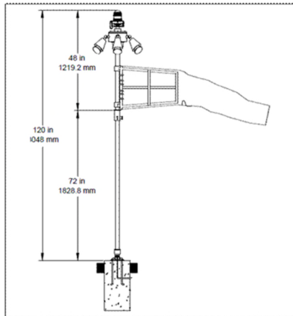
Figura 7-1. Instalación típica del indicador de la dirección del viento
