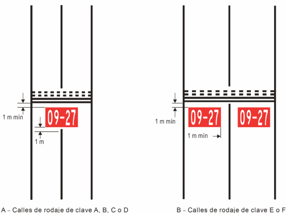
Figura 4-2-1. Señal con instrucciones obligatorias
