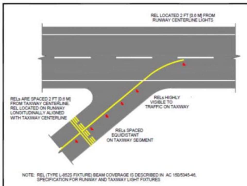
Figura 1-41-3 Sistema REL en ángulo
