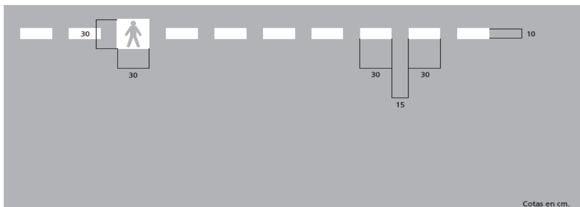
Figura 2-26-1. Señal de senda peatonal en Plataforma
