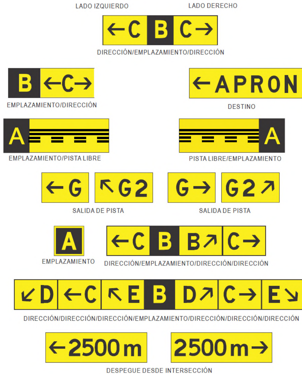
Figura 2-2-2. Letreros de información
