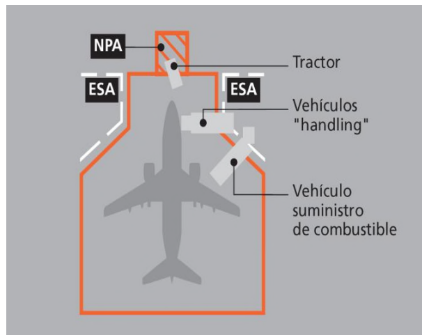
Figura 2-24-4. NPA delante del morro de la aeronave
