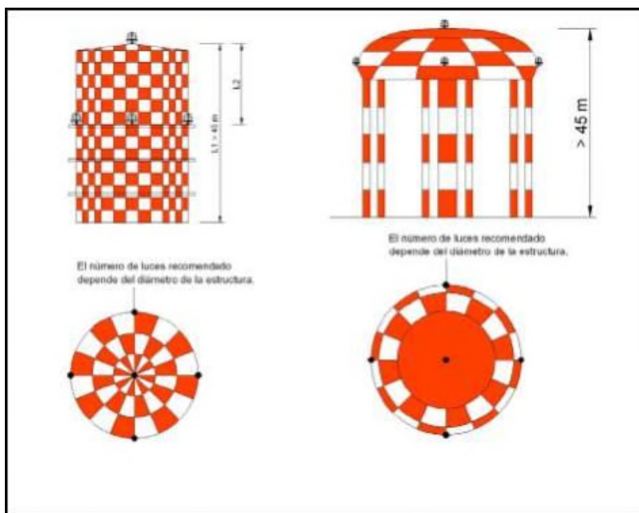
Figura 2-3-6. Ejemplos de iluminación de obstáculos/estructuras >45m
