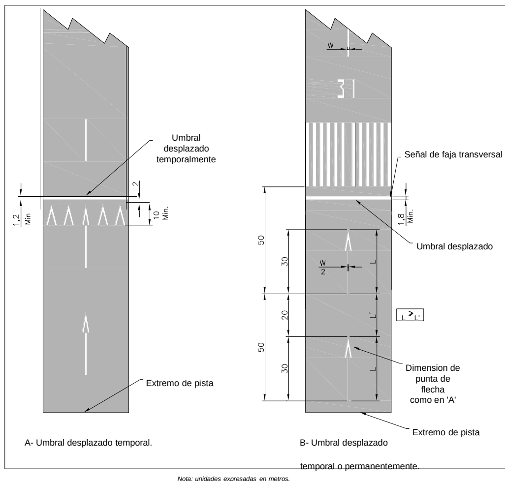
Figura 1-4-1. Señales de umbral desplazado
