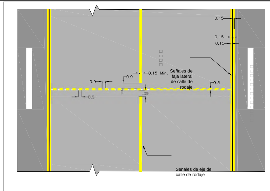
Figura 3-6-2. Señal de punto de espera intermedio.
