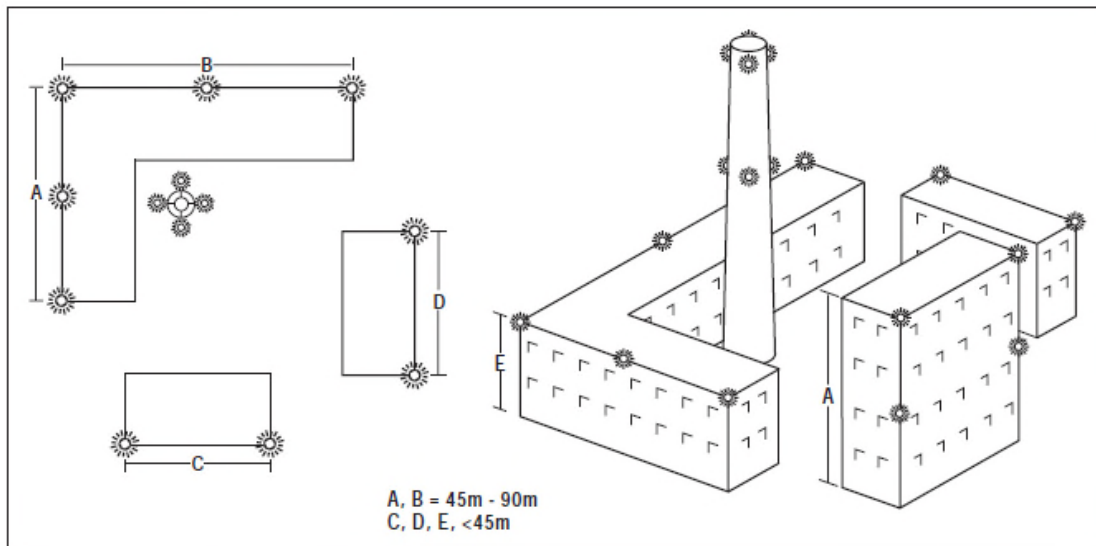
Figura 2-3-7. Ejemplos de iluminación de edificios
