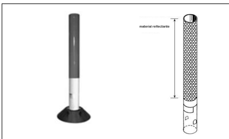
Figura 3-1 Balizas de borde de calle de rodaje
