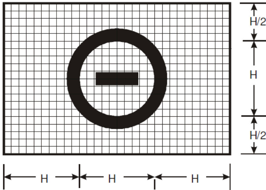
Figura ADJD-5. Ejemplo Letrero PROHIBIDA LA ENTRADA
