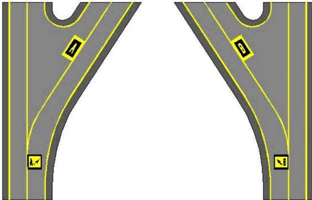
Figura 4-3-2. Señales de Información - emplazamiento
