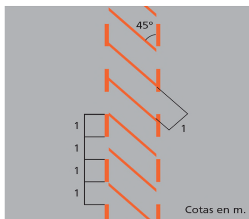
Figura 2-25-2. En caso de solape, la NPL será discontinua
