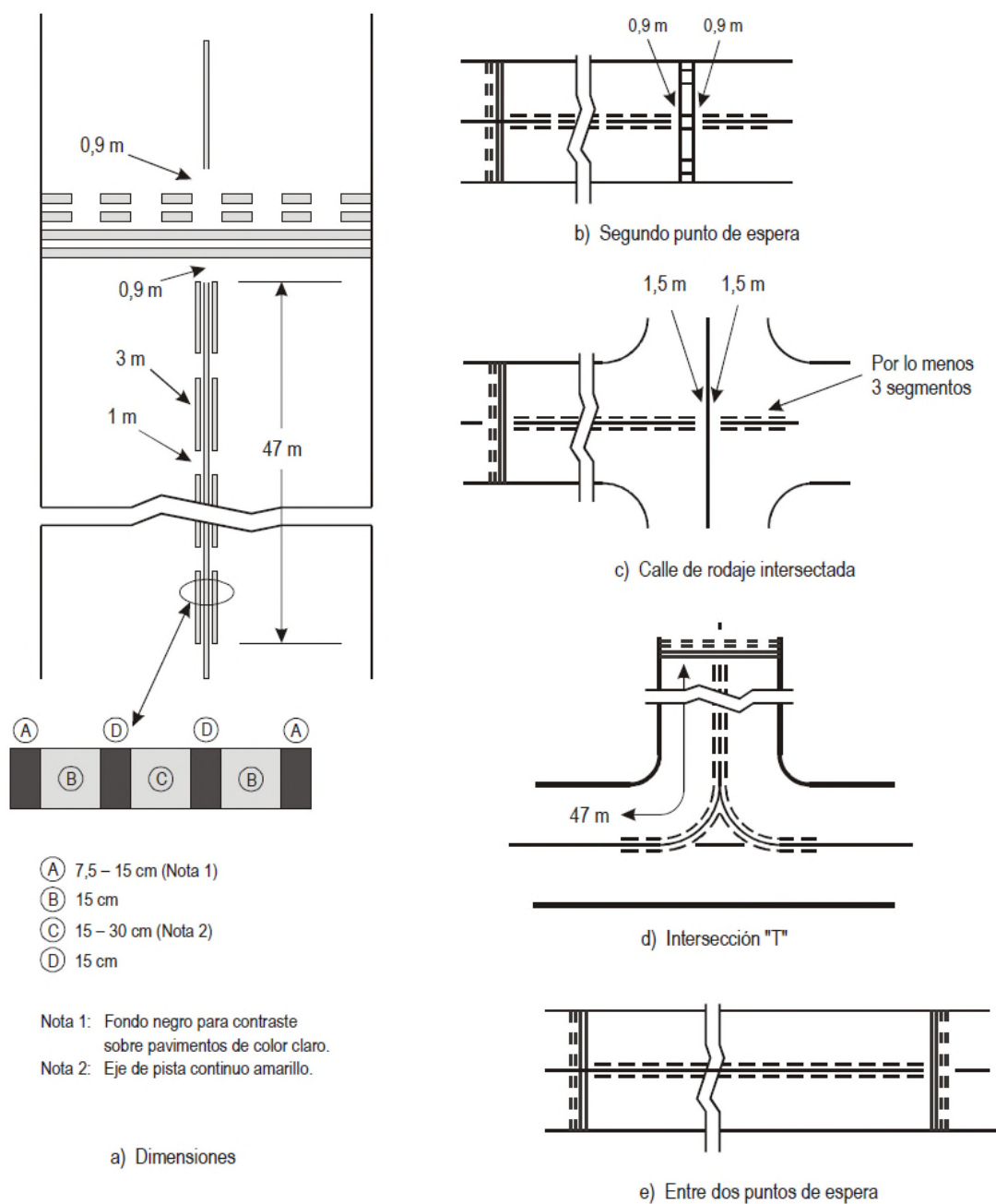
Figura 3-2-1. Señal mejorada de eje de calle de rodaje
