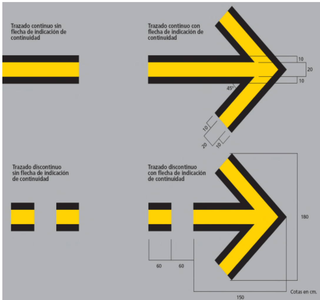
Figura 2-13-1. Señal de salida de puesto de estacionamiento
