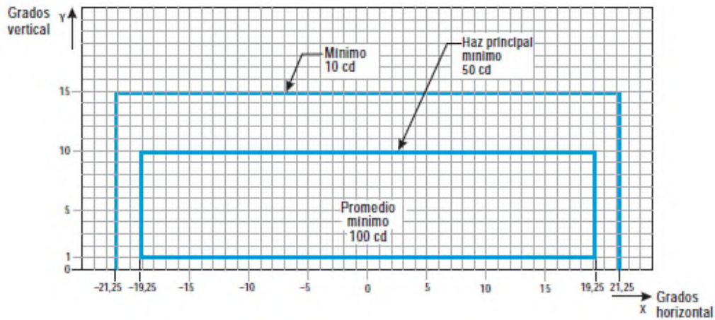
Figura ADJB-14. Diagrama de isocandelas para luces de eje de calle de rodaje (espaciado de 7,5 m), REL, de barra de prohibición de acceso y de barra de parada en tramos curvos para ser utilizado en condiciones de alcance visual en la pista inferior a un valor de 350 m
