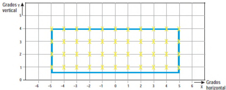
Figura ADJB-21. Puntos de cuadrícula para el cálculo de la intensidad media de luces de eje de calle de rodaje y de luces de barra de parada
