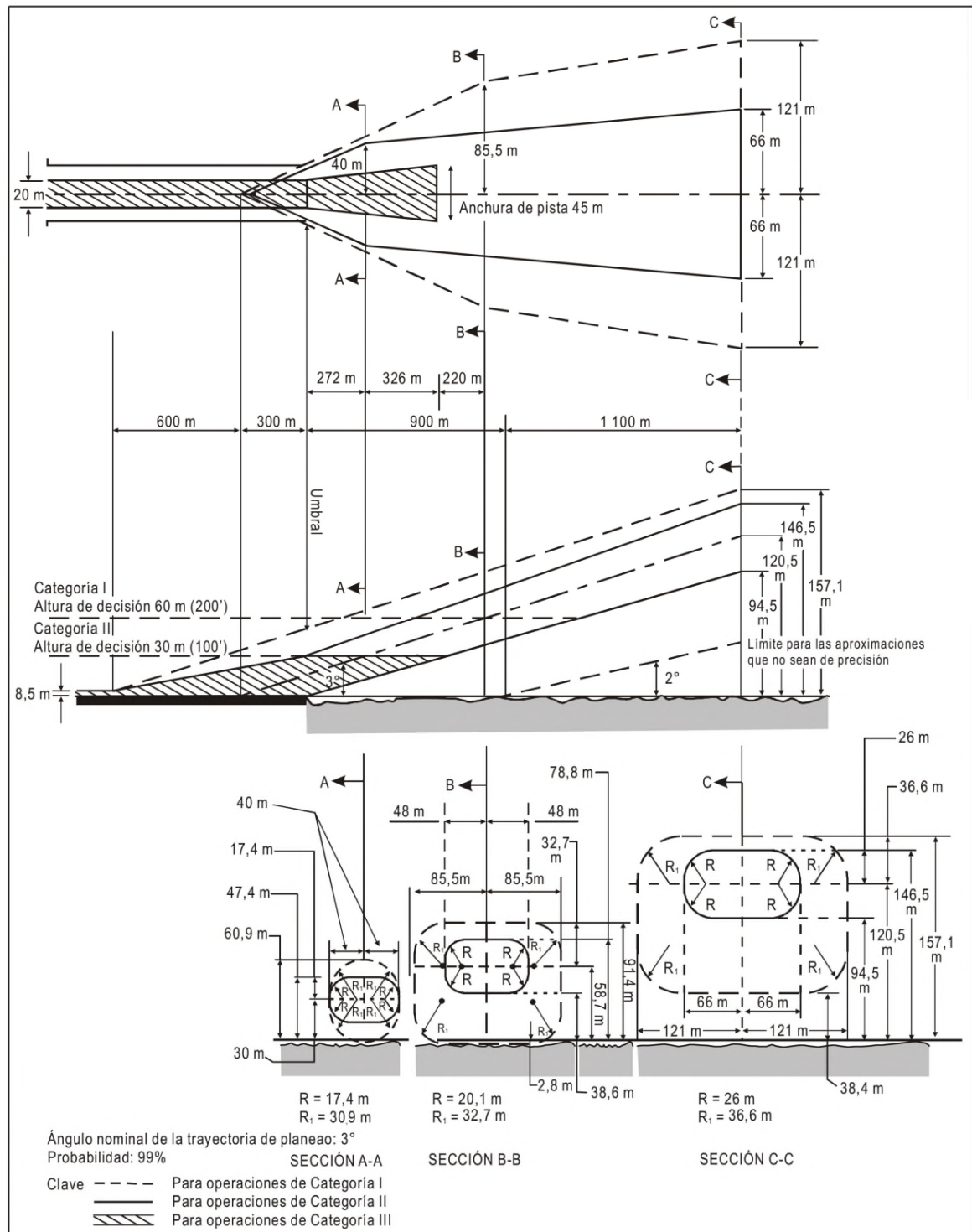
Figura ADJF-1. Envolventes de trayectorias de vuelo que han de utilizarse en el proyecto de iluminación para las operaciones de las Categorías I, II y III
