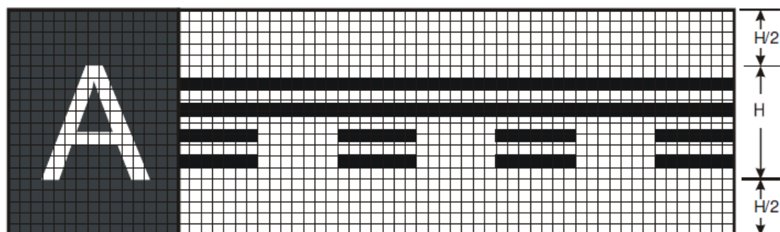
Figura ADJD-3A Ejemplo - Letrero de pista libre (con el letrero típico de emplazamiento)
