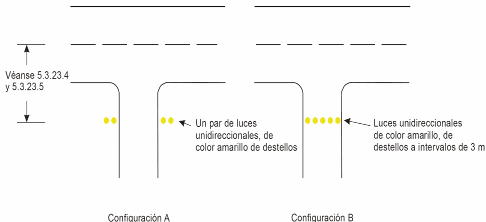
Figura 1-31-1. Luces de protección de pista
