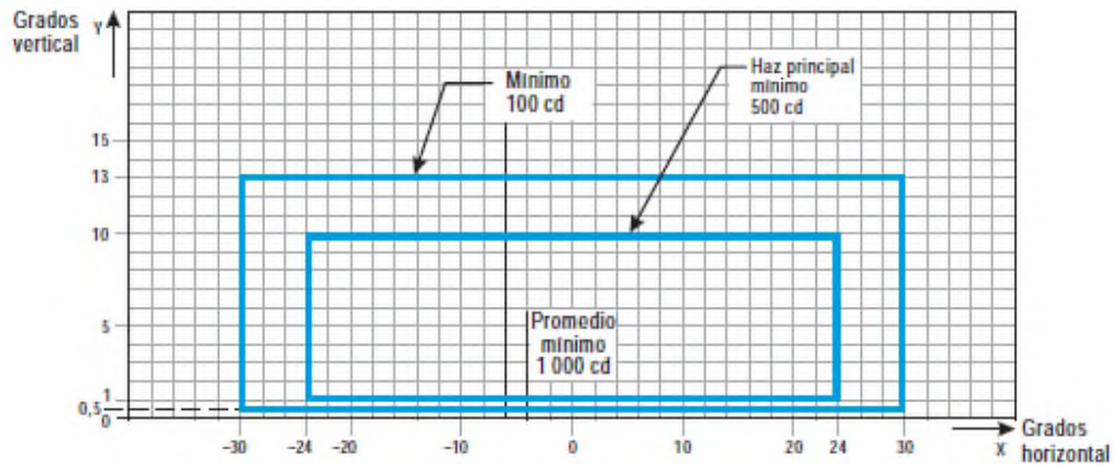
Figura ADJB-20. Diagrama de isocandelas para las luces de protección de pista de alta intensidad, configuración B
