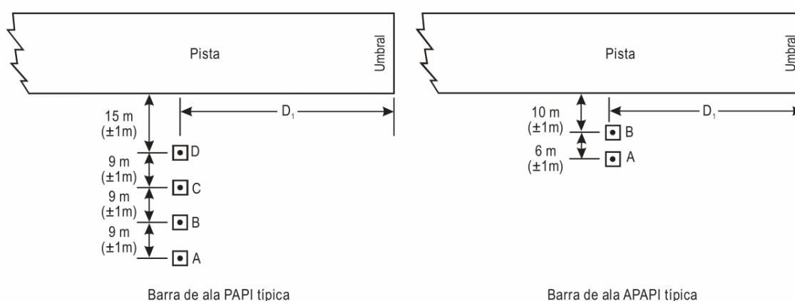
Figura 1-9-3. Emplazamiento del PAPI y APAPI
