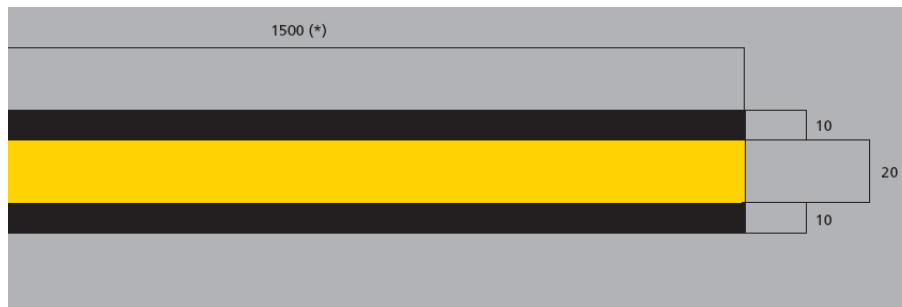
Figura 2-19-1. Señal de Barra de alineación
