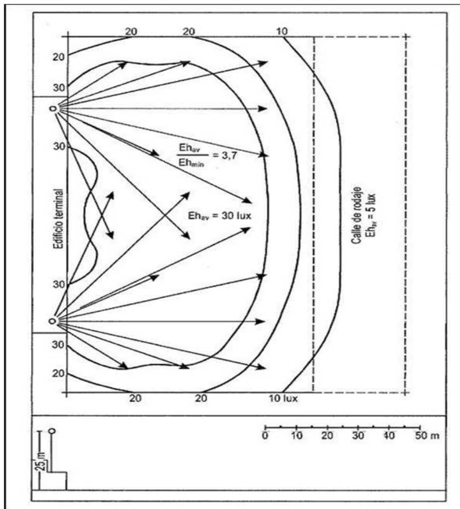
Figura ADJM-3 Curvas características de isolux para luminancia horizontal (Ejemplo A)
