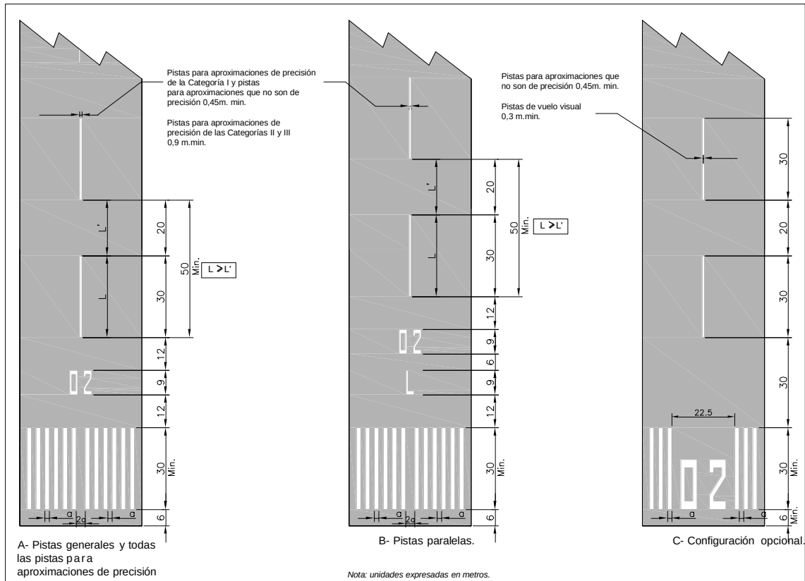
Figura 1-3-1. Señales de designación de pista, de eje y de umbral
