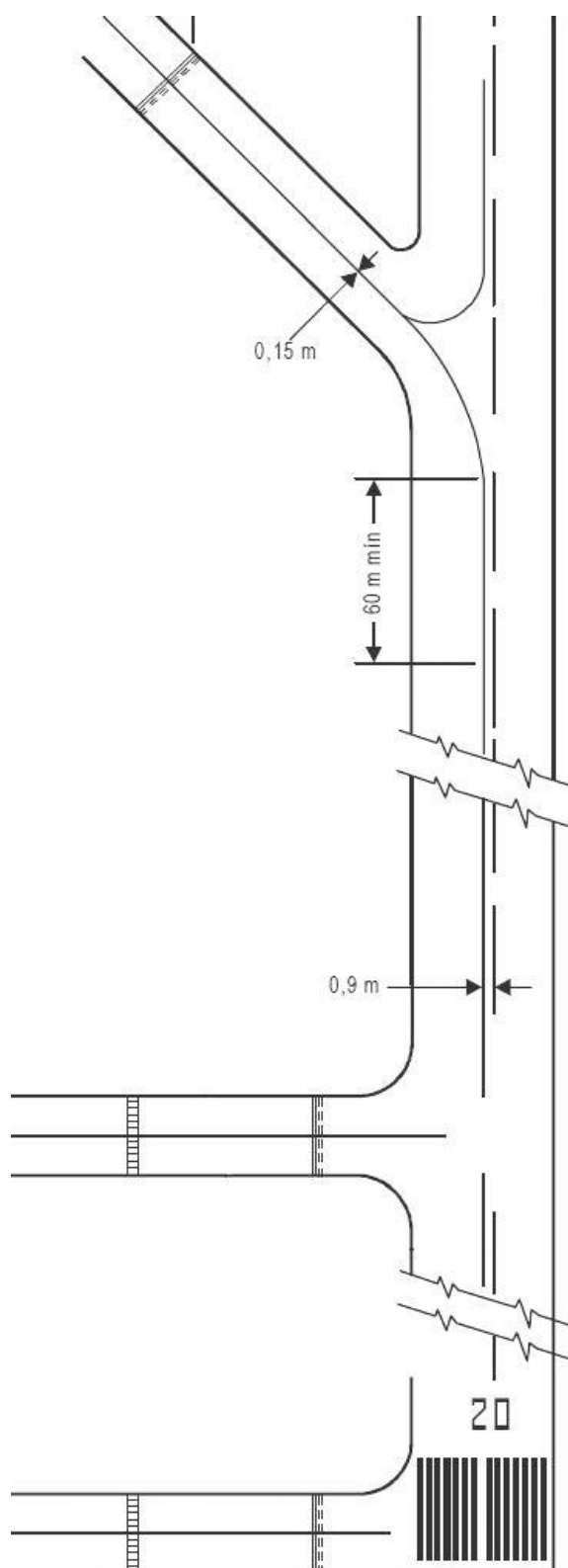
Figura 3-1-1. Señal de eje de calle de rodaje
