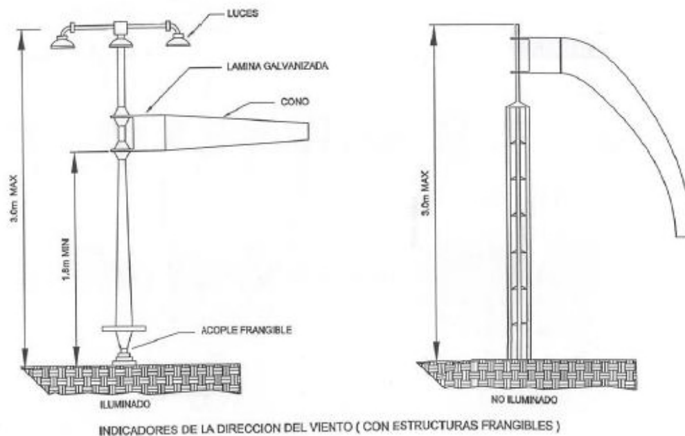
Figura 7-2. Estructuras frangibles
