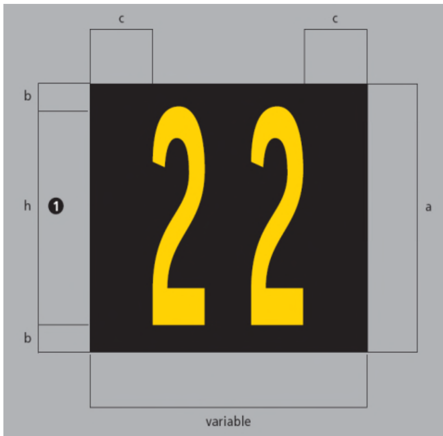
Figura 2-18-1 Señal de designación del puesto de estacionamiento
