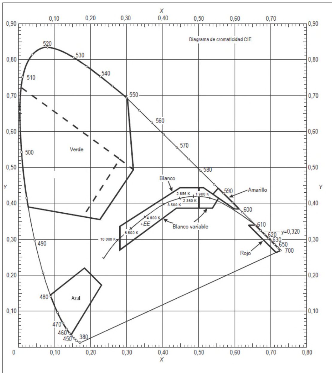
Figura ADJA-2-1a. Colores de luces aeronáuticas de superficies (lámparas de tipo filamento)
