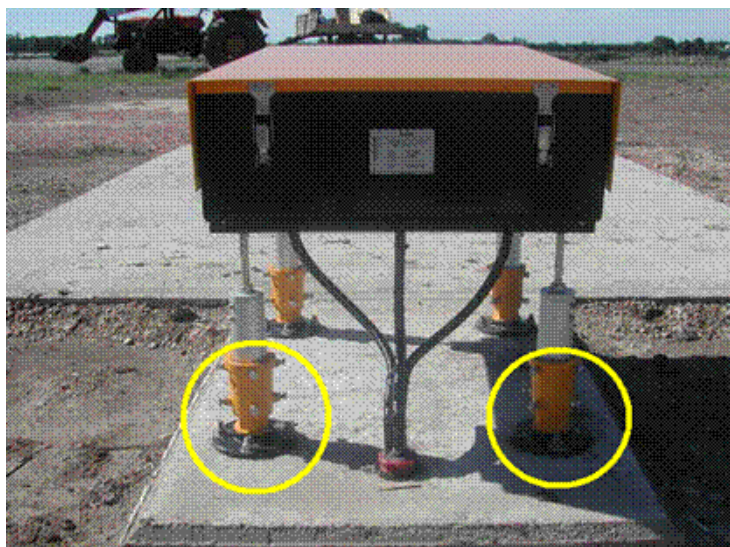
Figura 2-6-5. Ejemplos de cuplas Frangibles en las instalaciones del PAPI
