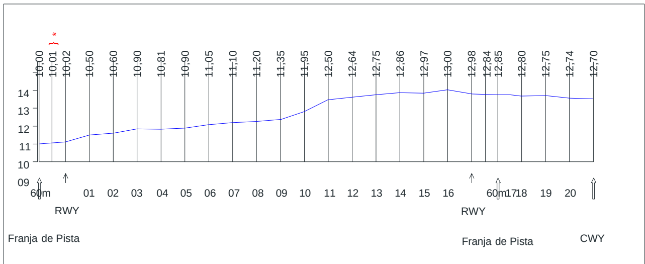
Figura 6-20 – Información contenida en la Planta del Perfil Longitudinal Acotado
