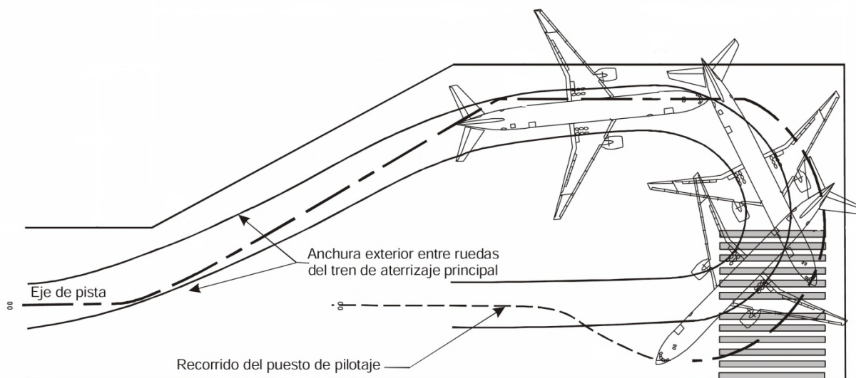
Figura 3-4-3. Ejemplo del recorrido de la aeronave en la plataforma de viraje
