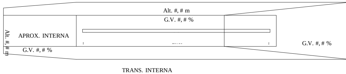
Figura 6-16 - Superficie de Aproximación Interna, Transición Interna y Aterrizaje Interrumpido
