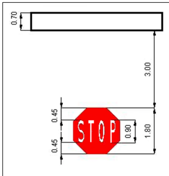
Figura 4-1-1 Señal de detención. Características y emplazamiento
